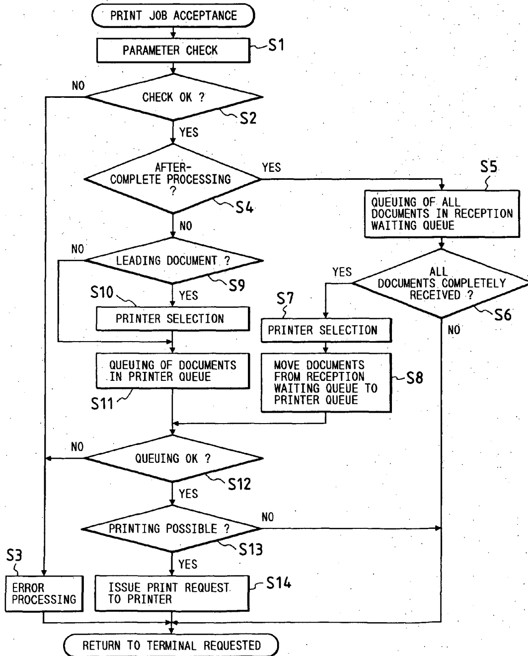
FIG. 31
