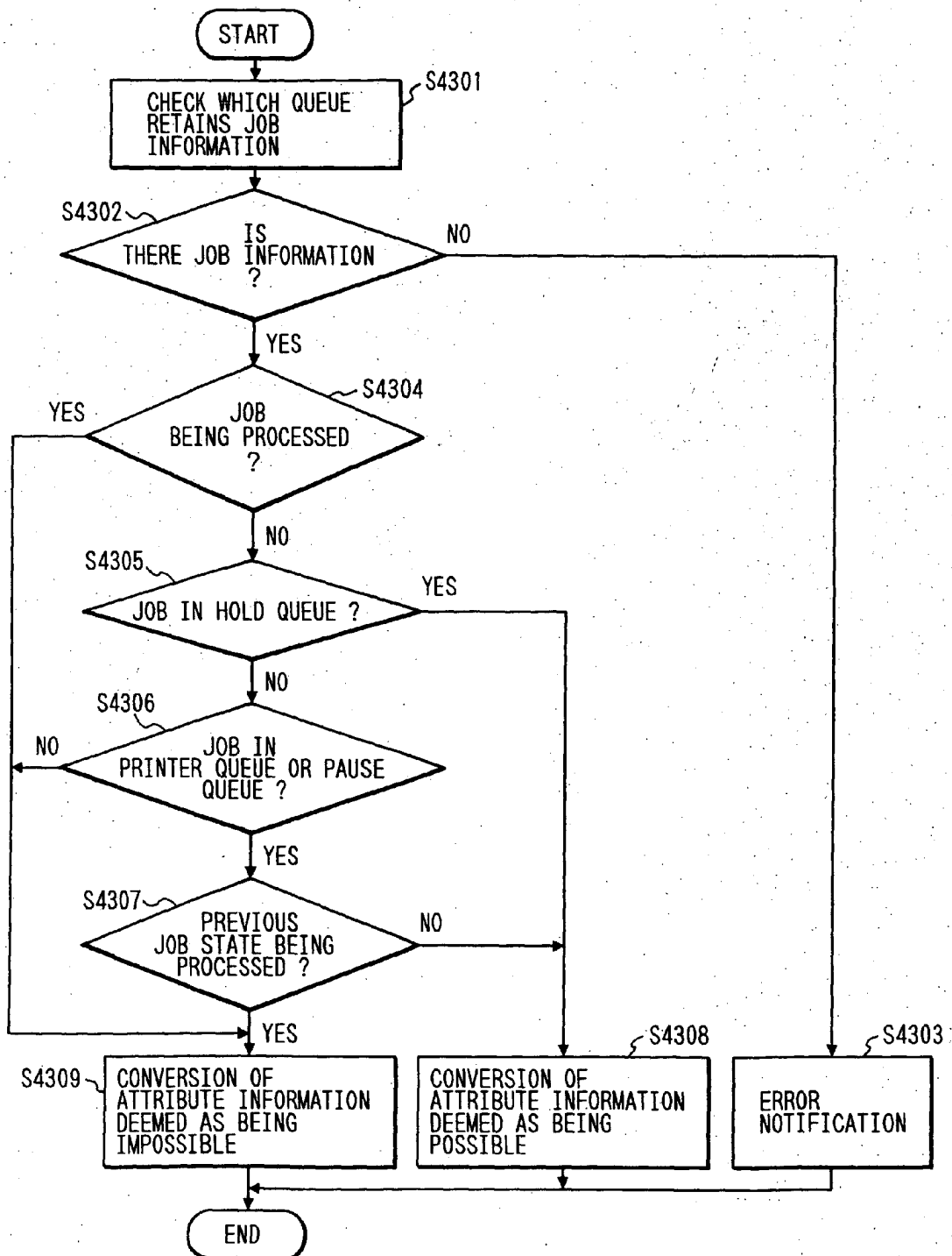
FIG. 46
