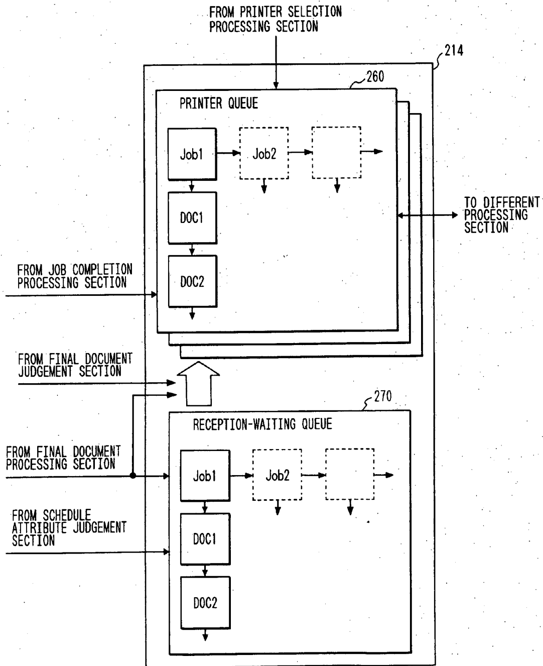
FIG. 29
