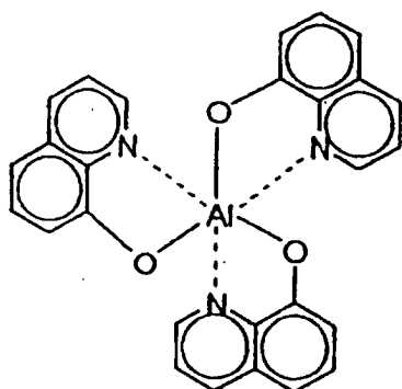
Alq3
