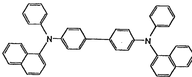
\alpha -NPD
