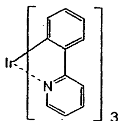
Ir(ppy) 3
