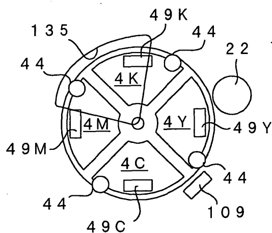
FIG. 37 A: HOME POSITION
