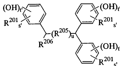
(D7)
