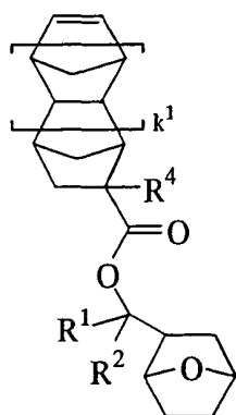
(3)
