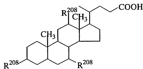
(D14)
