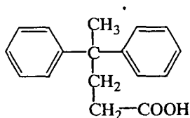
(AII-4)
