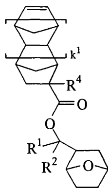
(3)
