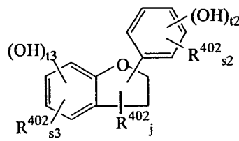
(A9)
