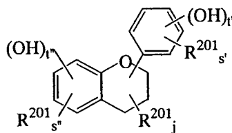
(D10)
