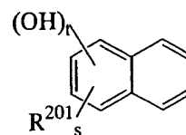
(D3)
