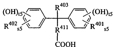
(A11)
