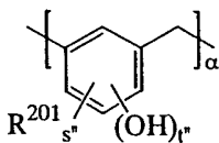
(D9)
