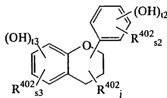
(A8)
