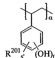
(D8)
