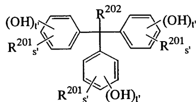
(D5)
