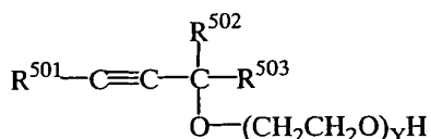
(S1)
