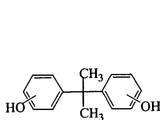
(D1)
