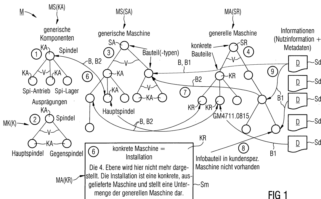
Bild 1: Maschinenbasismodelle
