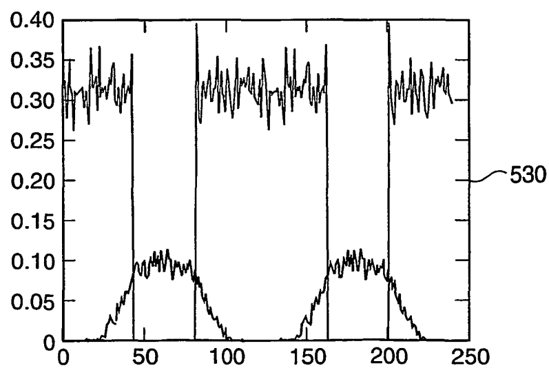
FIG. 5c 0.01 Torr
