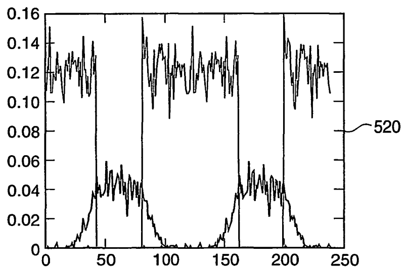
FIG. 5b 0.1 Torr
