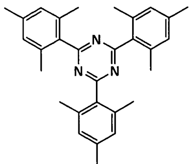
D1-1
