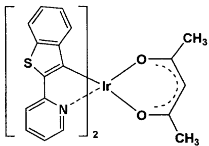
Ir-9
