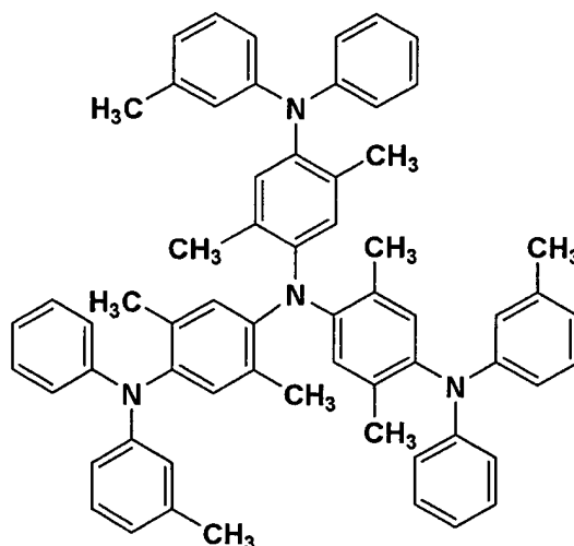
m-MTDATXA
