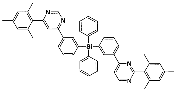
A1-5
