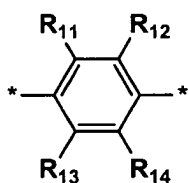
formula (d)
