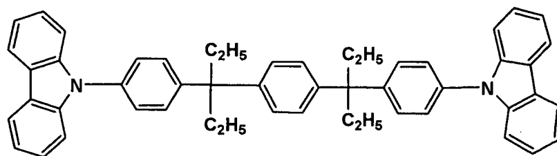
HA-7
