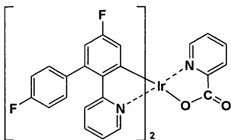
Ir-13
