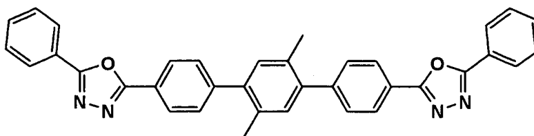
A1-1
