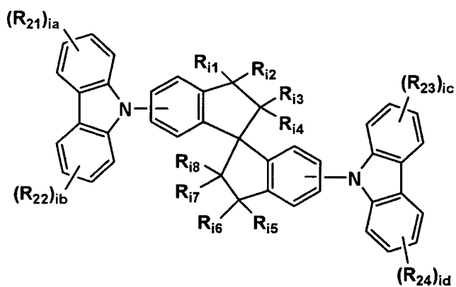
Formula I1
