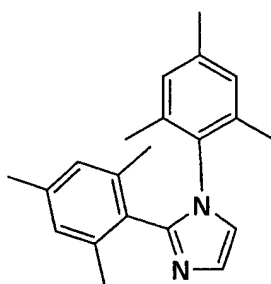
F1-2
