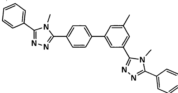
A1-3
