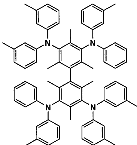
C-21
