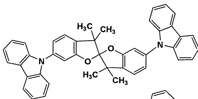
JA-5
