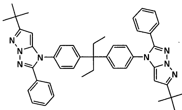
A3-3
