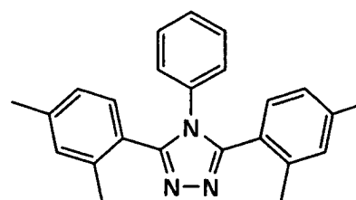
B1-2
