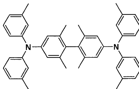
C-2
