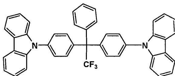
HC2
