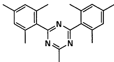
D1-3
