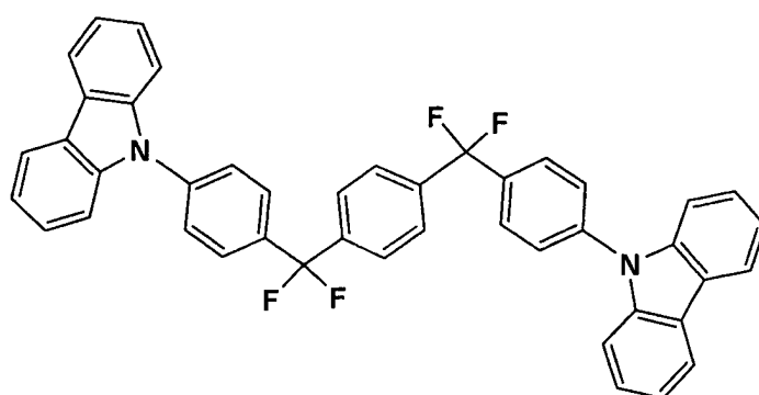
12-42
