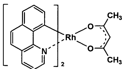
D-5
