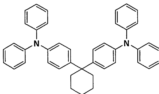
C-3
