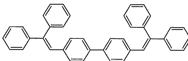
(DPVBi)
