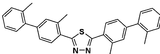
E1-1
