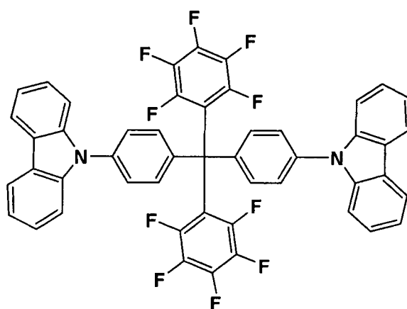
HC7
