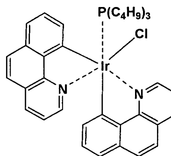
Ir-6
