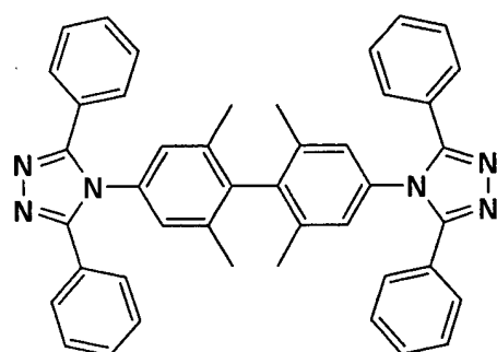
A2-2
