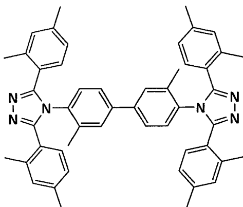
A2-3
