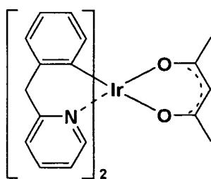
D-3
