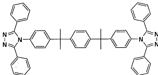
A1-7
