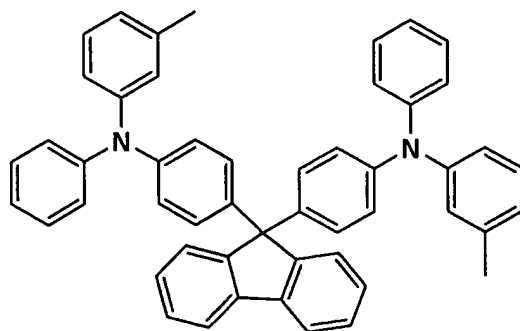
C-16
