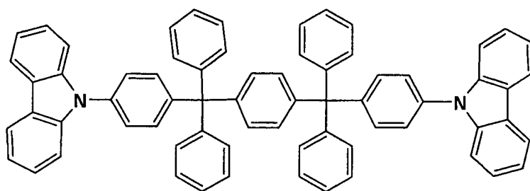
HC10
