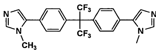
A1-4
