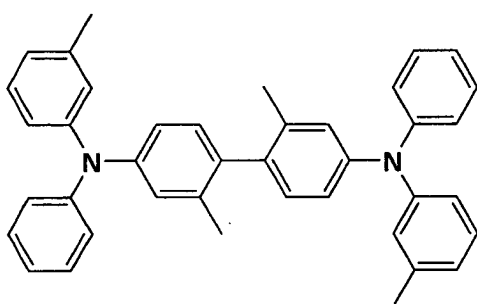
C-1
