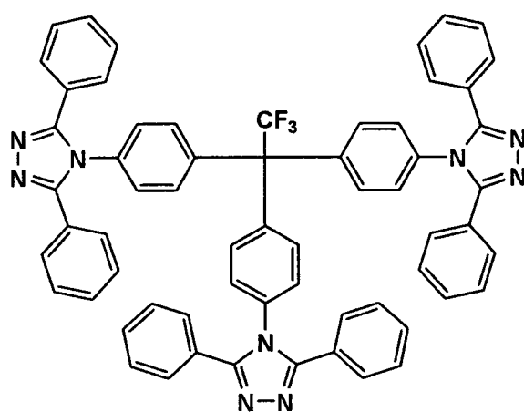
A3-2
