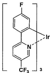
D-1
