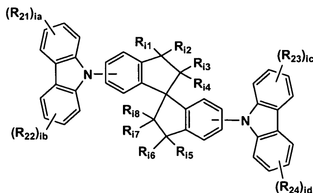
Formula I1
