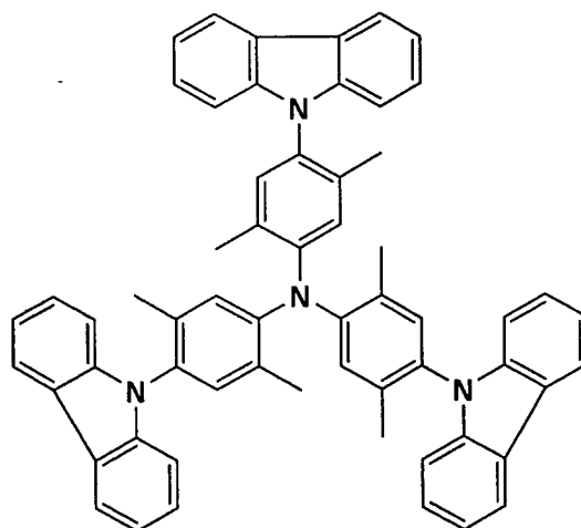
C-6
