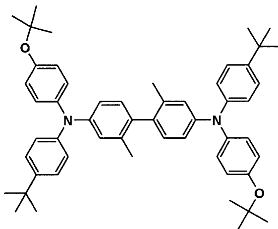
C-22
