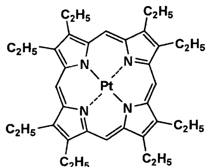
Pt-3
