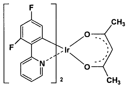
Ir-10
