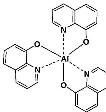
Alq 3
