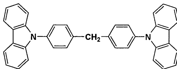
14-1
