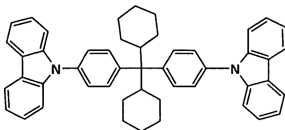
HC1
