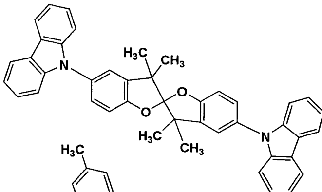
JA-7
