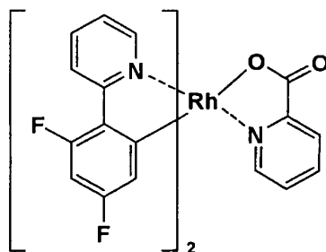
Rh-2
