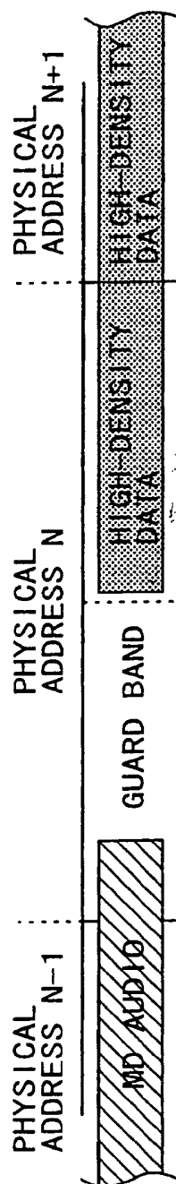
FIG. 21A
