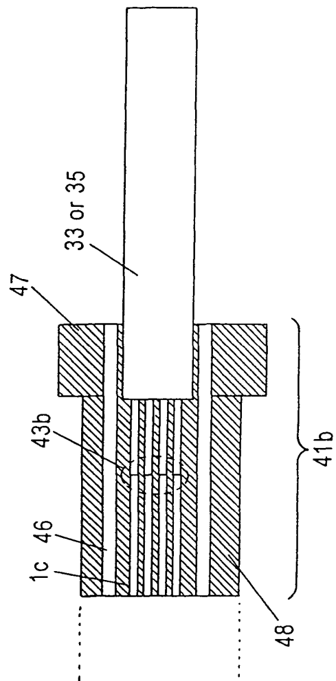
FIG. 10A
