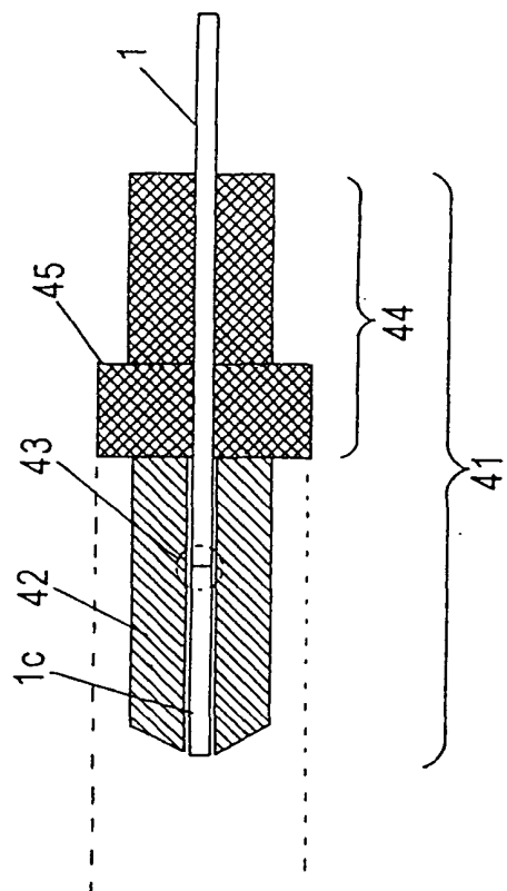
FIG. 9A
