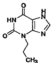
Enprofylline
