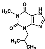
1-Methyl-3-isobutylxanthine
