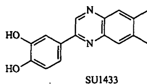
SU1433
