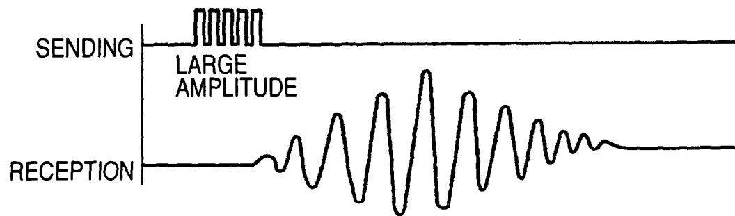
FIG. 13B
