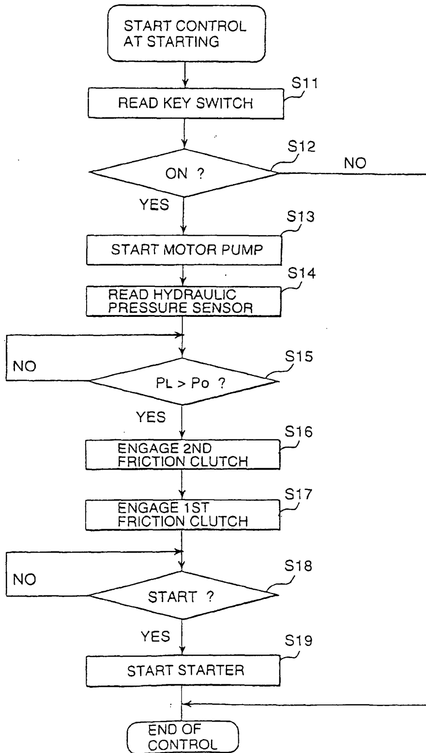
FIG. 8B
