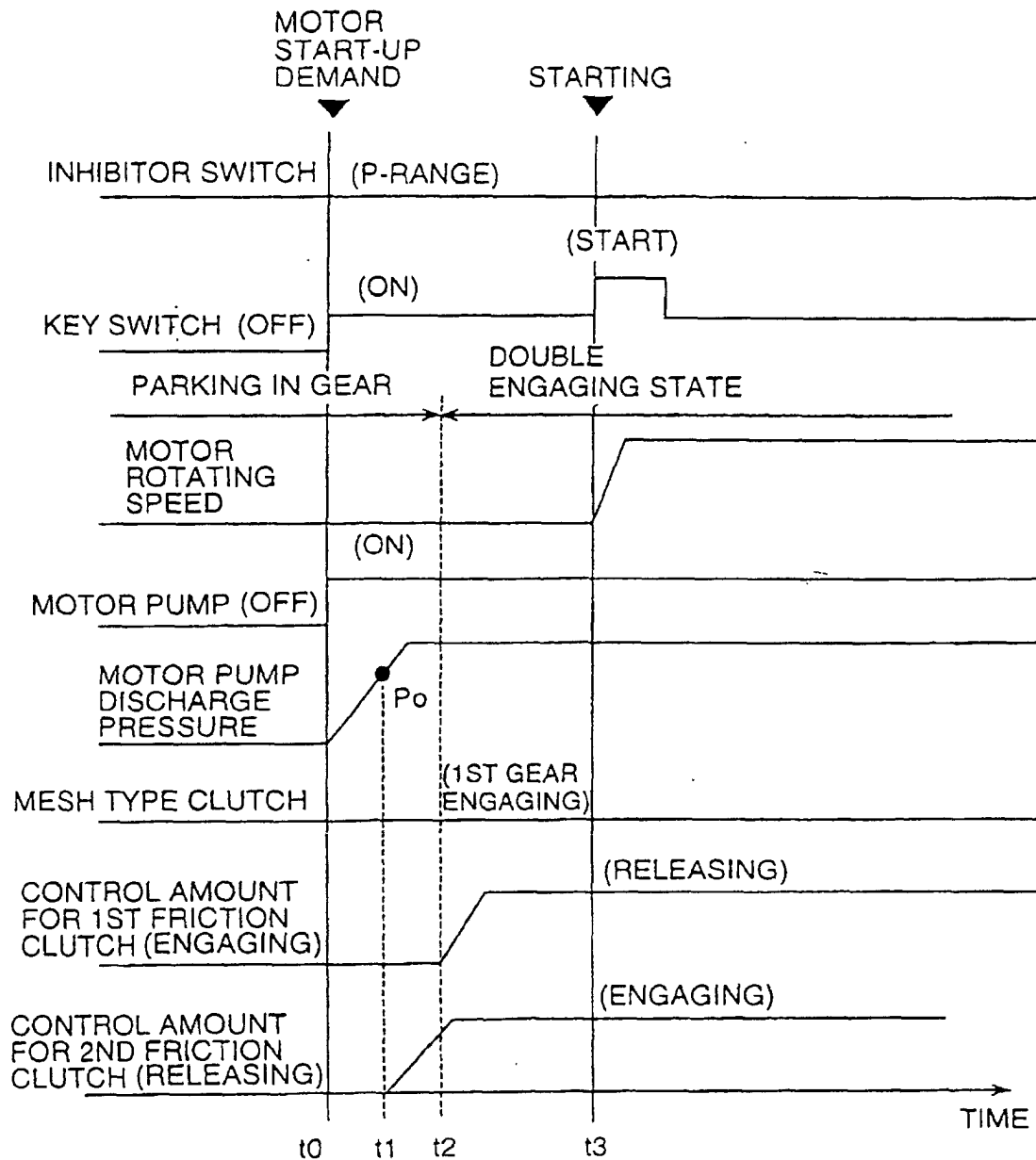
FIG. 9B
