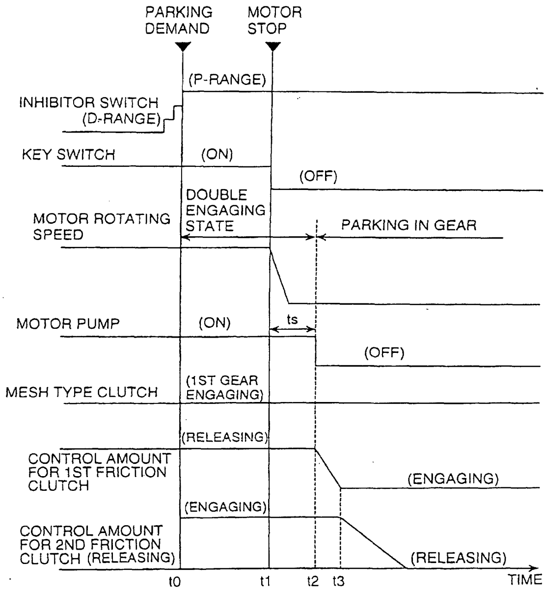
FIG. 9A
