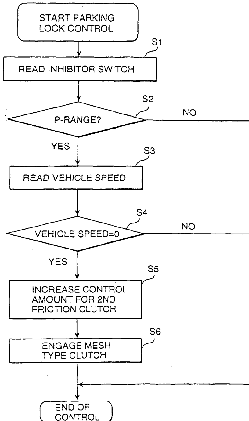
FIG. 8A
