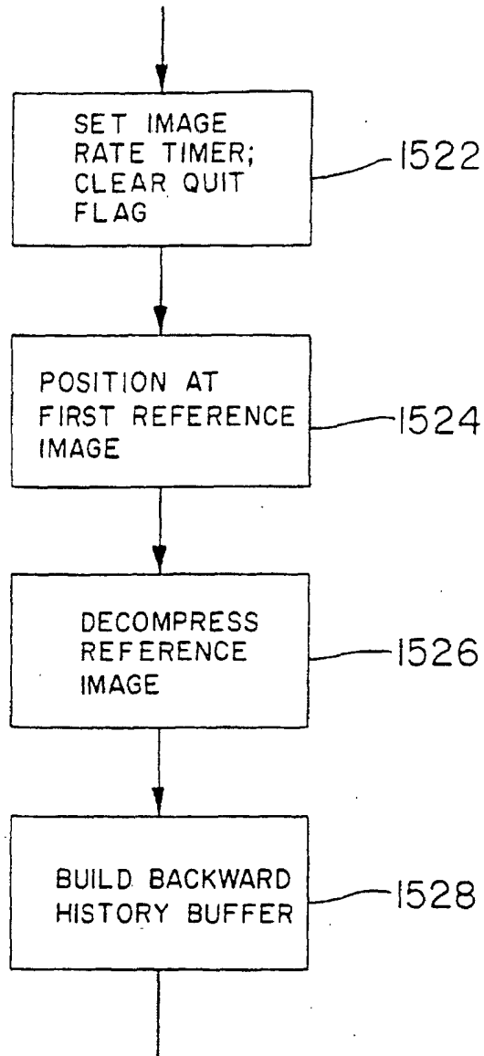
FIG. 65A BACKWARD DECOMPRESSION
