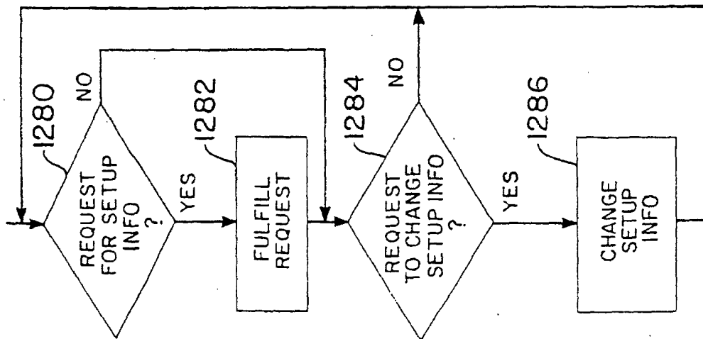
FIG. 50 SETUP MGR.
