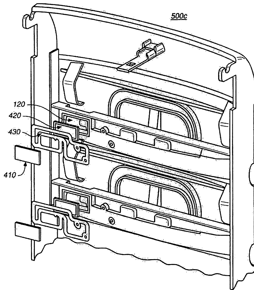
FIG. 5C
