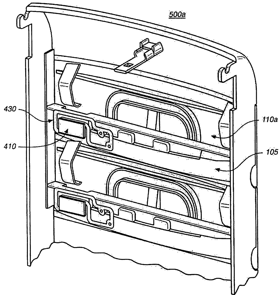
FIG. 5A
