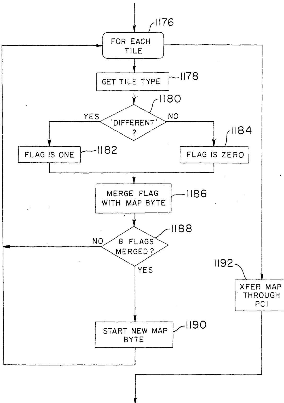
FIG. 39A MAP GENERATOR
