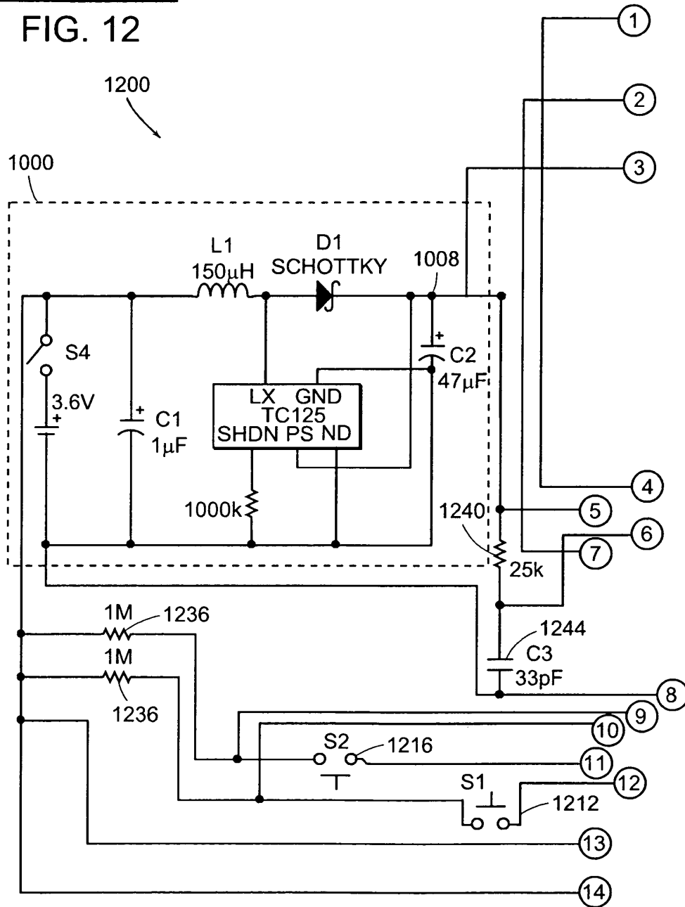
FIG. 12A
