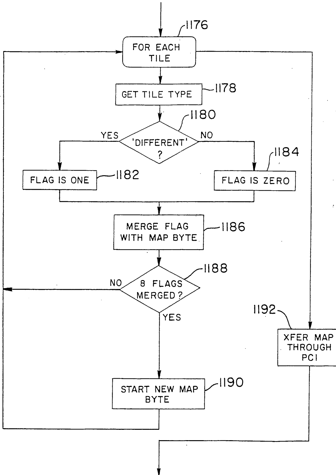
FIG. 39A MAP GENERATOR
