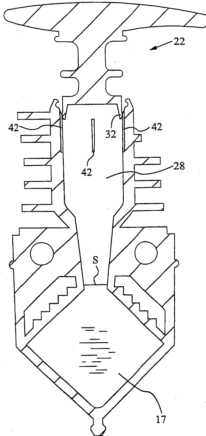
FIG. 7B
