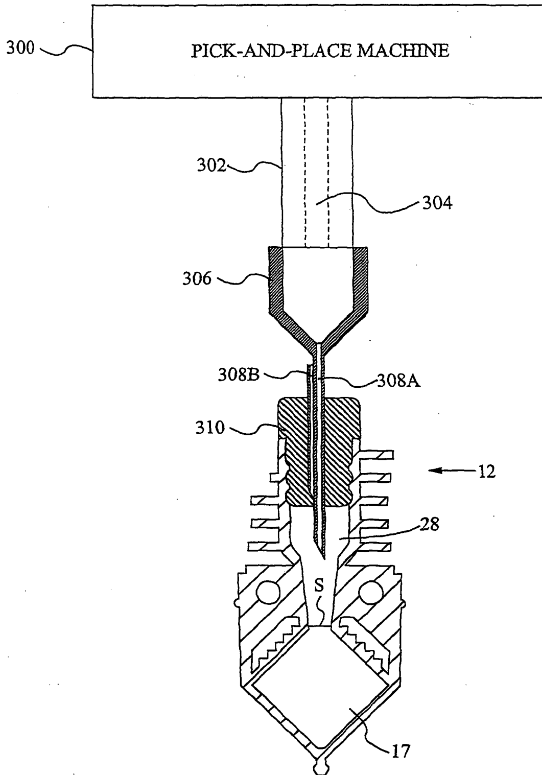
FIG. 35
