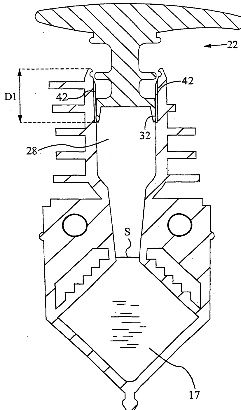
FIG. 7C
