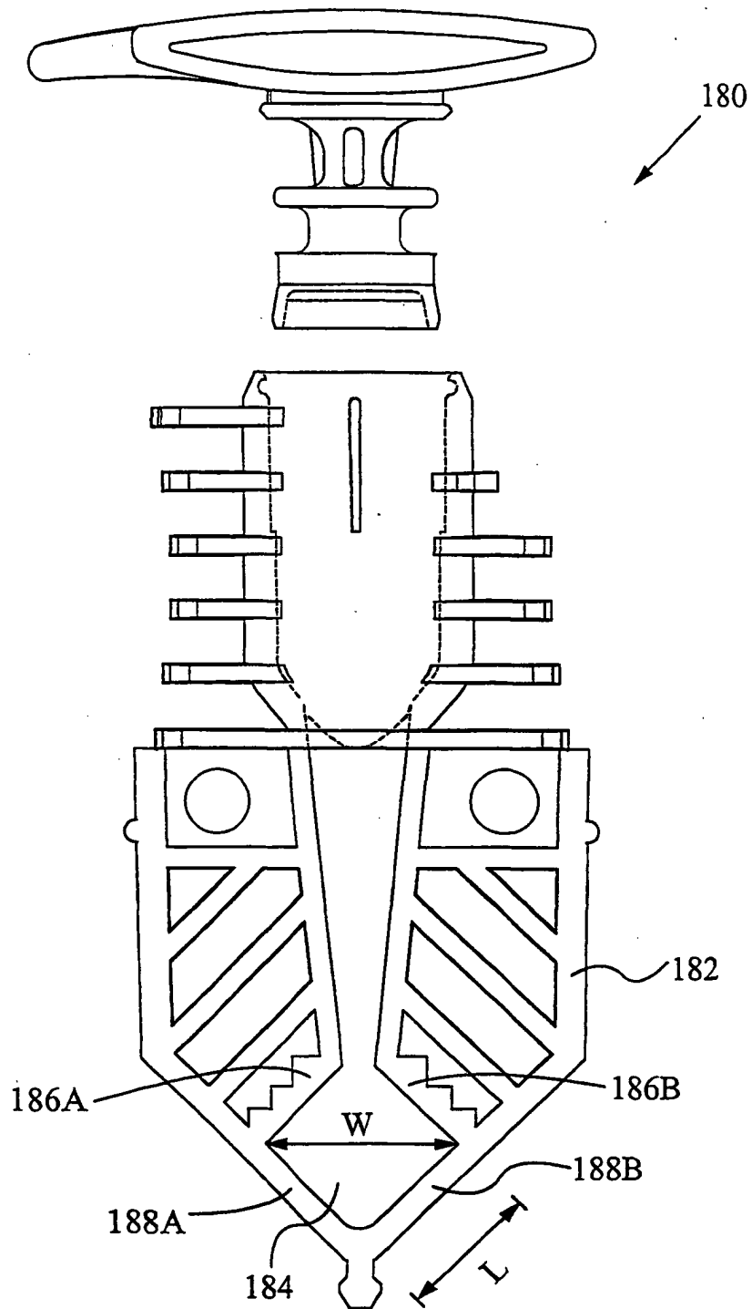
FIG. 26
