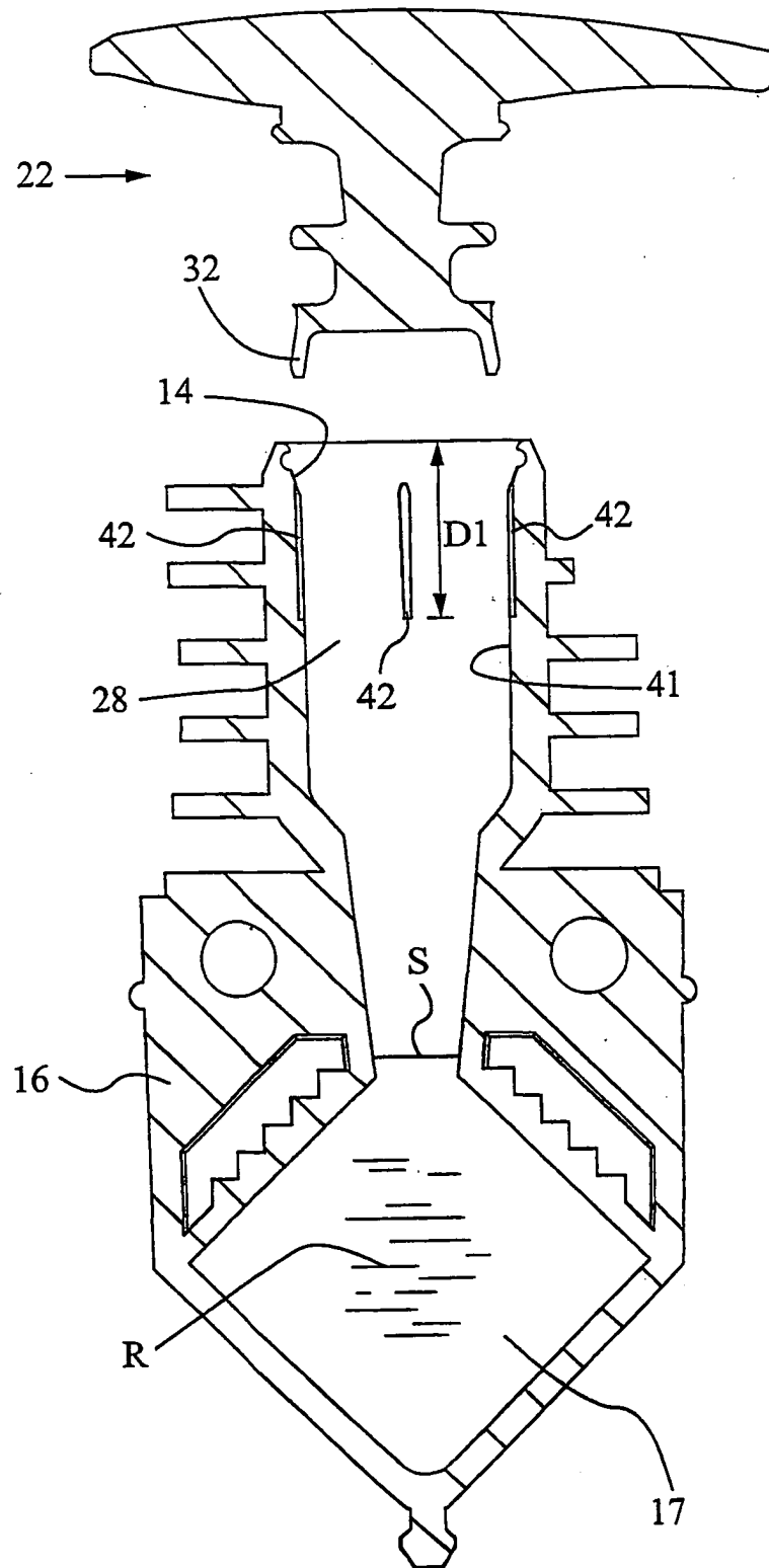
FIG. 7A
