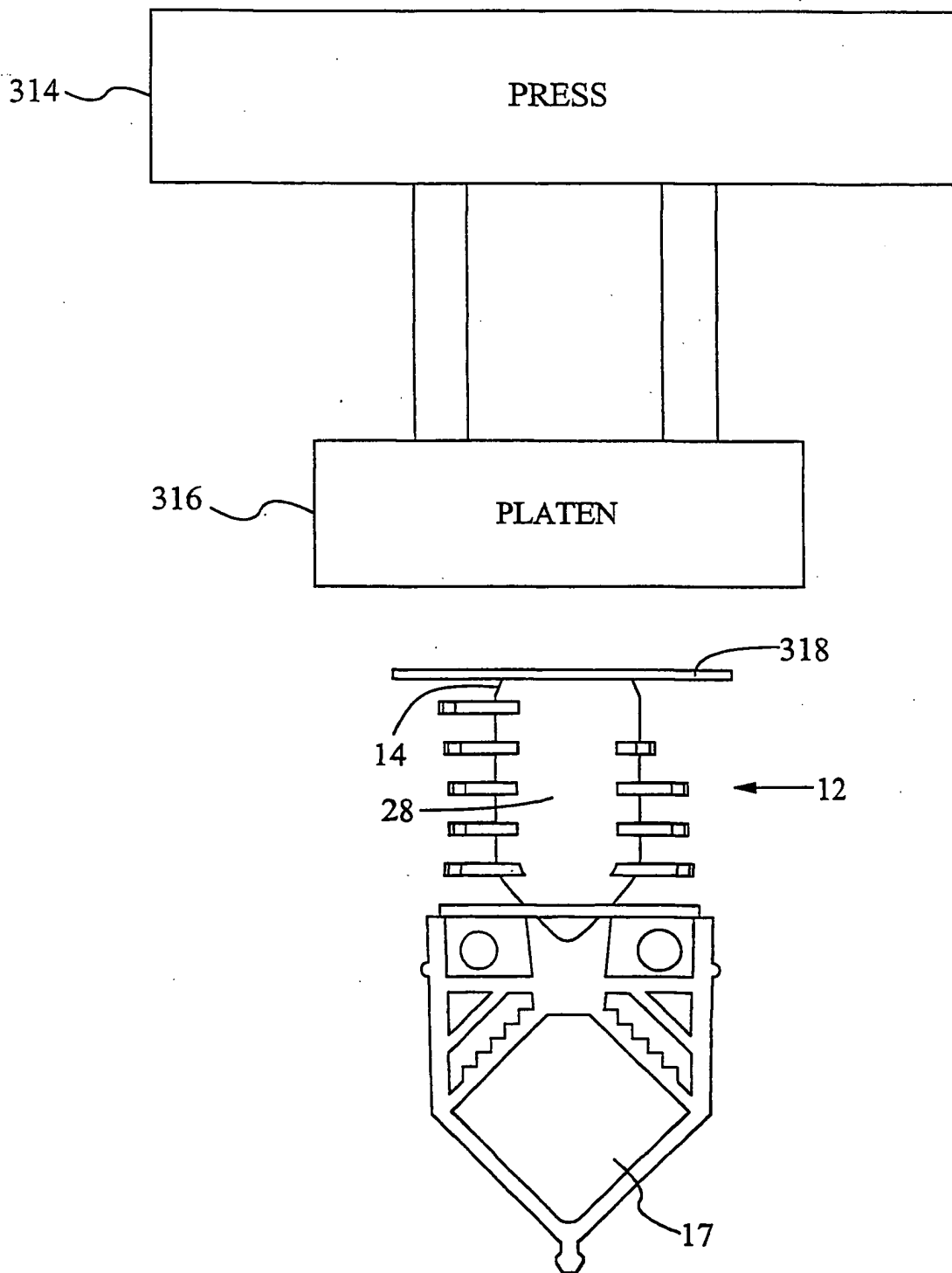
FIG. 38
