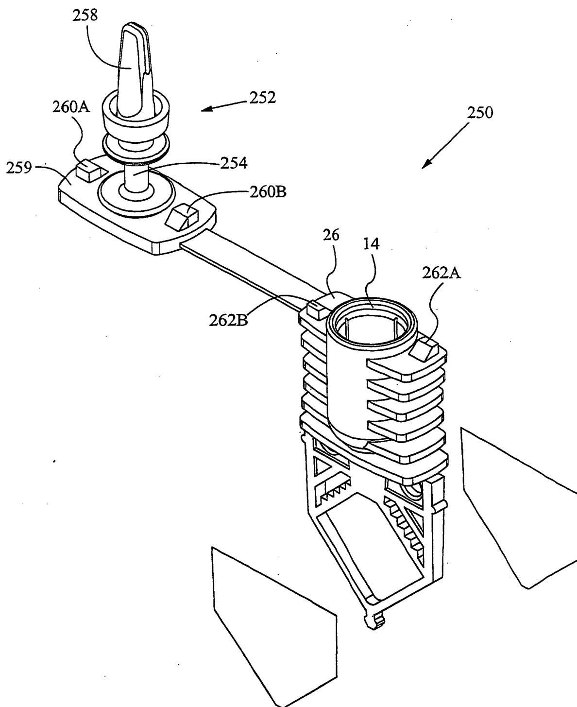
FIG. 28
