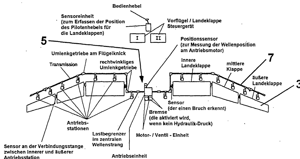
Fig. 1 Stand der Technik Landeklappensystem A 340
