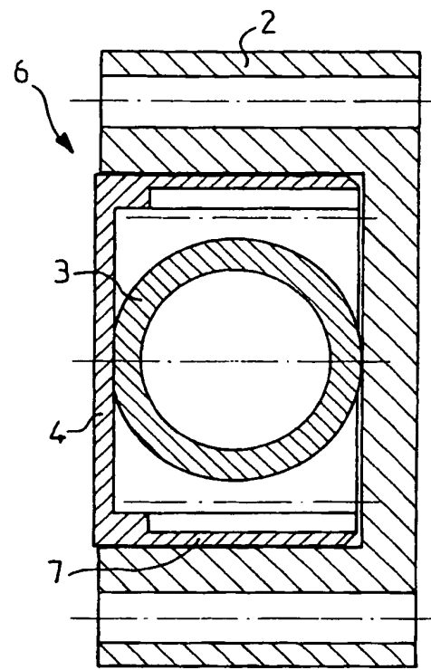
FIG. 9 A-A
