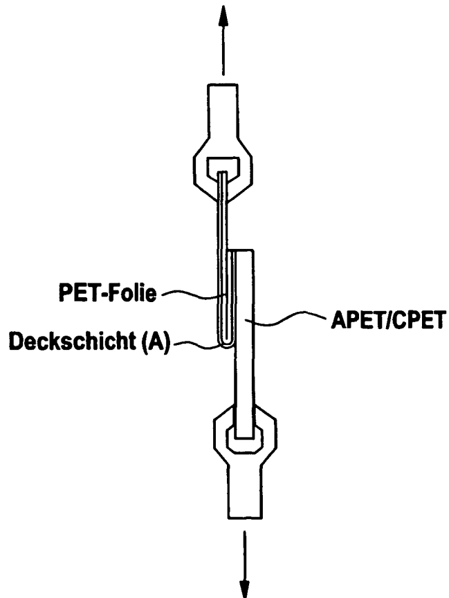
Fig. 2 Anordnung von "peelfähiger" Folie und Streifen einer APET/CPE-Menueschale im Zug-Dehnungs-Messgerät
