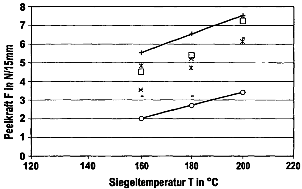
Fig. 5 Zusammenhang zwischen Siegeltemperatur in °C und Peelkraft in N/15mm
