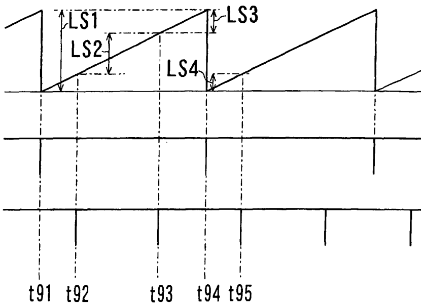
FIG. 34A (LS)
