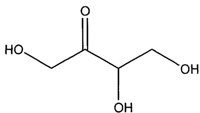
Erythrulose
