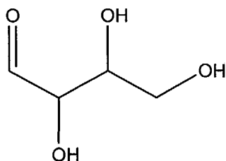
Erythrose
