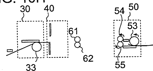
FIG. 10H
