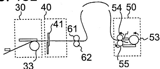
FIG. 10E
