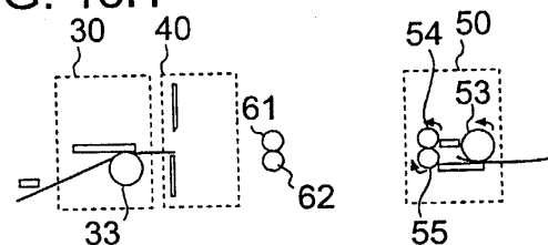
FIG. 13H
