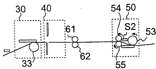
FIG. 13F
