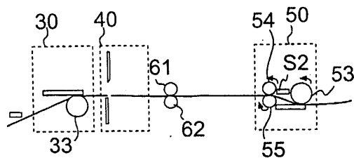
FIG. 10G
