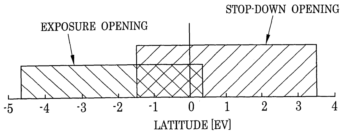
FIG.9B
