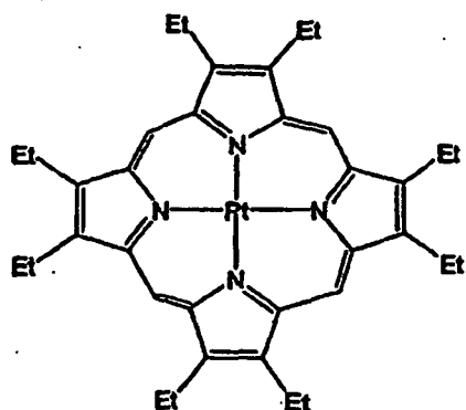
PtOEP
