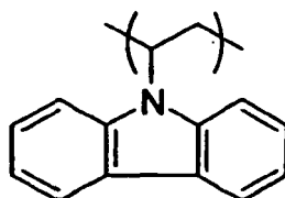
PVK
