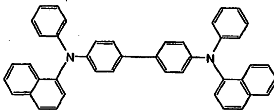
\alpha -NPD
