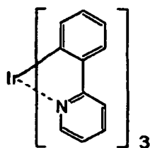
Ir(ppy) 3
