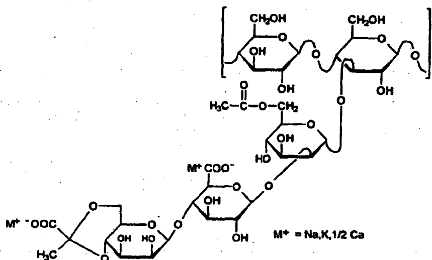
Grundeinheit von Xanthan
