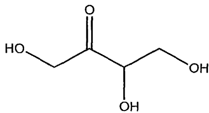
Erythrulose
