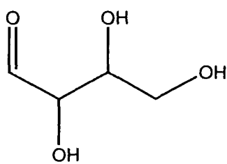
Erythrose
