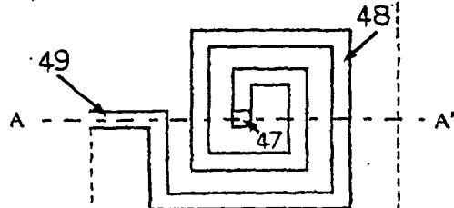
Fig. 4 (d) Top view of the fourth layer
