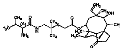
1-Valnémuline
