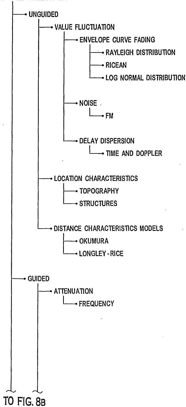
FIG. 8A
