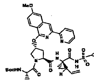
Verbindung 320
