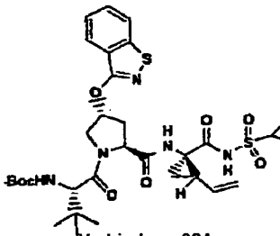
Verbindung 324
