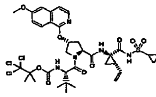
Verbindung 68
