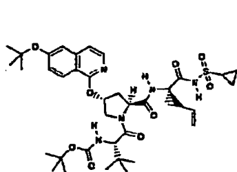
Composé 193 ;
