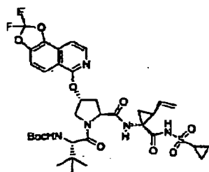
Verbindung 287
