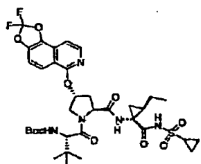
Composé 289 ;
