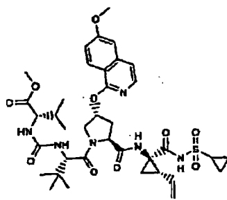
Verbindung 141
