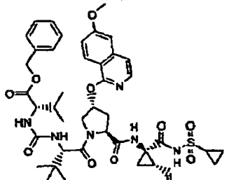
Verbindung 150
