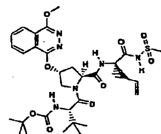
Composé 201
