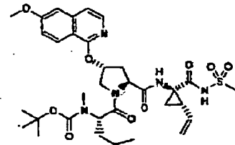
Composé 86
