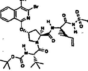
Verbindung 224
