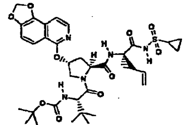
Verbindung 211
