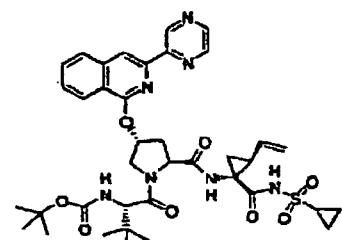
Verbindung 31
