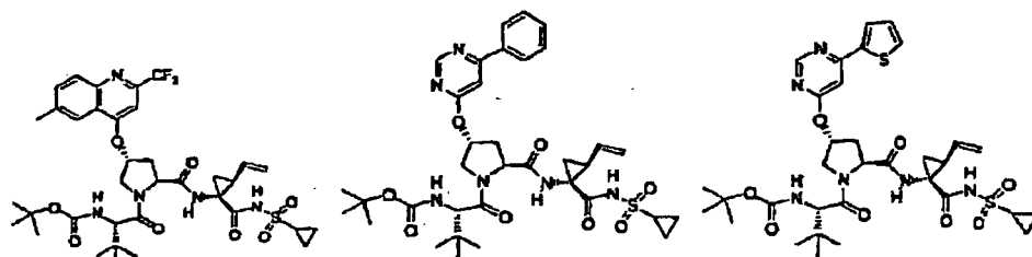
Composé 410 ;
