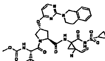
Verbindung 341
