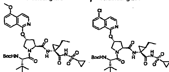
Verbindung 292
