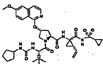
Composé 75
