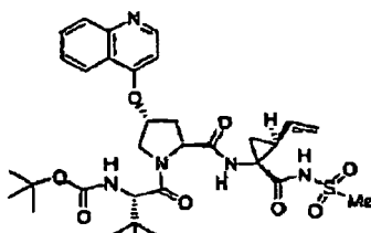
Verbindung 386
