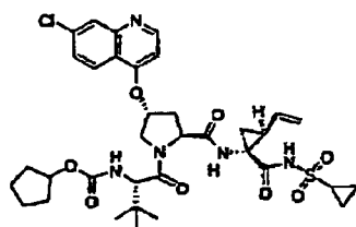
Composé 372
