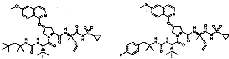
Verbindung 81
