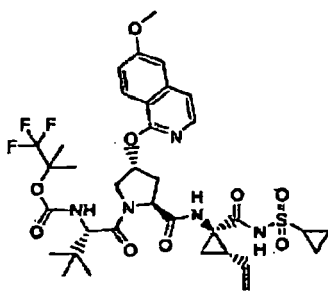
Verbindung 155
