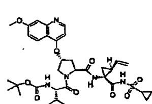
Composé 378 ;
