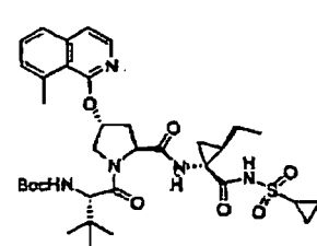
Composé 297 ;
