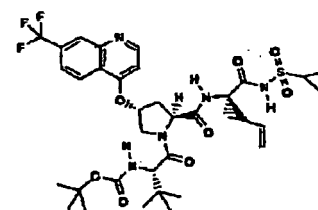
Verbindung 185
