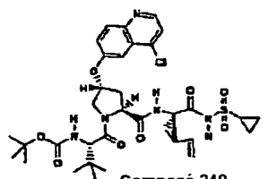
Composé 240
