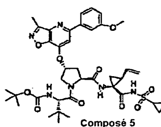
Composé 5
