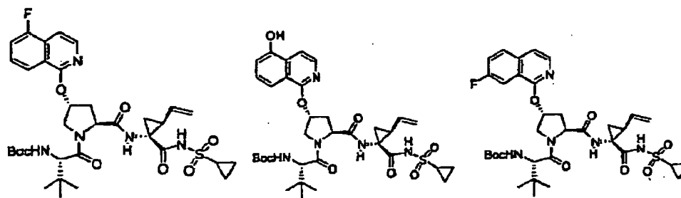
Verbindung 257
