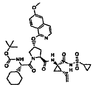
Composé 143
