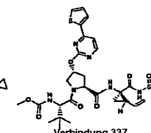
Verbindung 337
