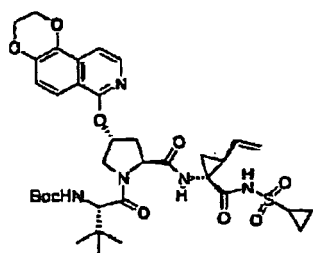
Verbindung 286
