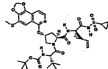
Verbindung 213
