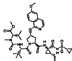
Verbindung 154
