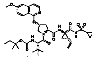
Verbindung 67
