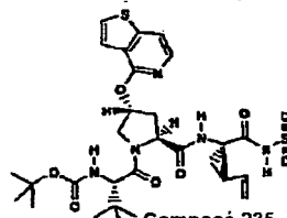
Composé 235
