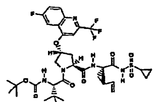
Verbindung 238
