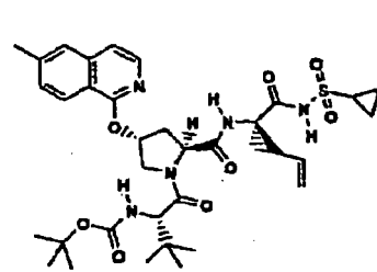
Composé 210 ;
