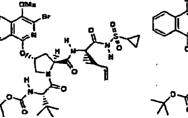
Verbindung 223
