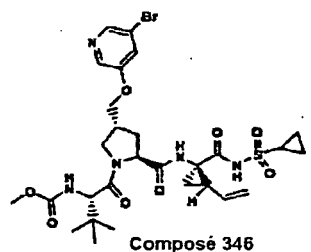
Composé 346
