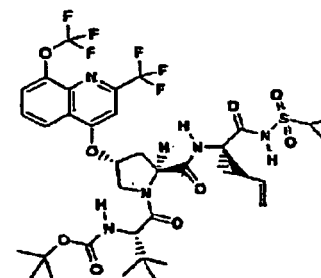
Composé 182
