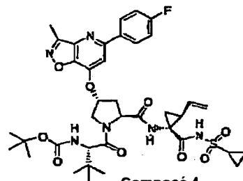
Composé 4
