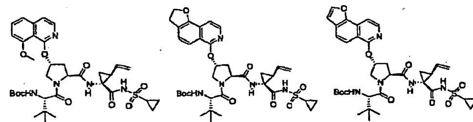
Verbindung 266
