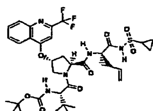
Verbindung 180
