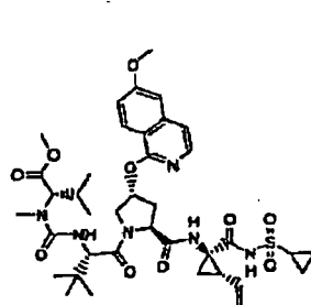
Composé 154
