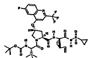
Composé 238
