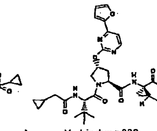
Verbindung 339
