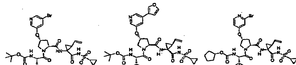
Composé 424 ;
