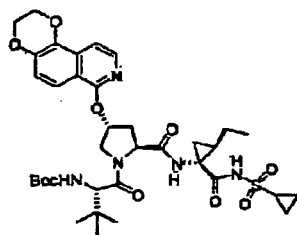
Verbindung 290
