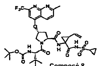
Composé 8
