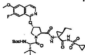
Composé 298
