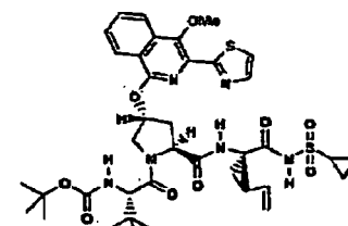
Verbindung 232
