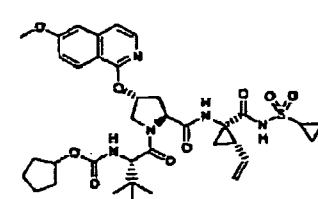
Verbindung 70
