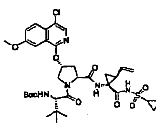
Verbindung 284
