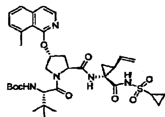
Verbindung 263
