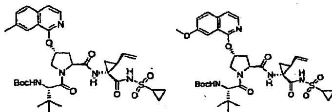
Verbindung 260
