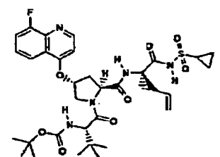
Composé 241
