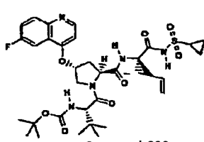
Composé 239
