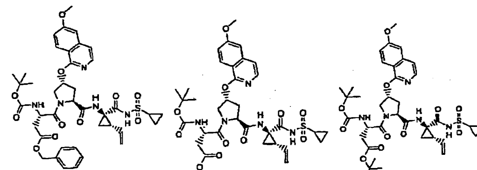
Verbindung 137
