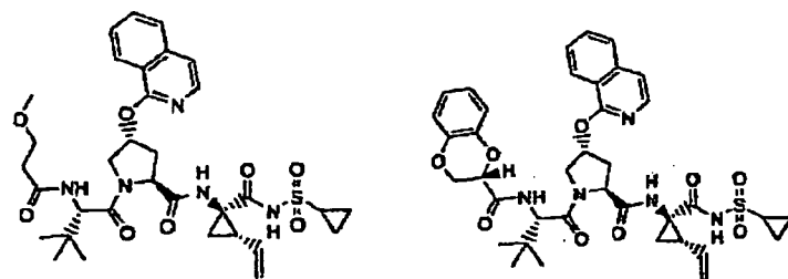
Verbindung 132
