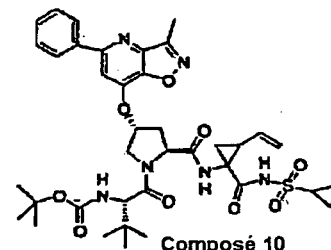
Composé 10
