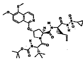
Composé 207 ;
