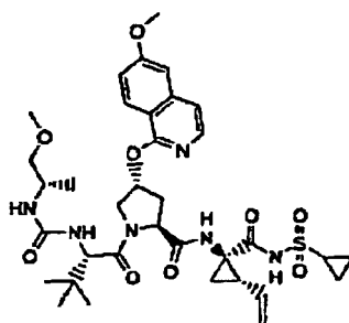
Verbindung 153
