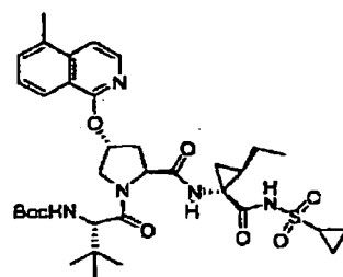
Verbindung 293
