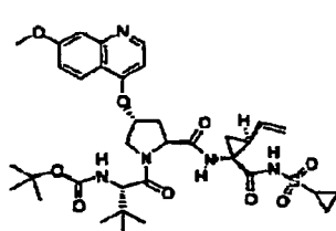
Verbindung 376
