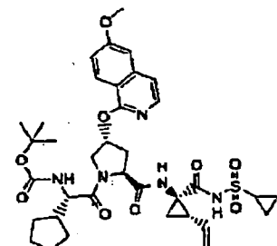
Verbindung 149
