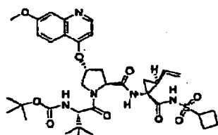
Verbindung 374
