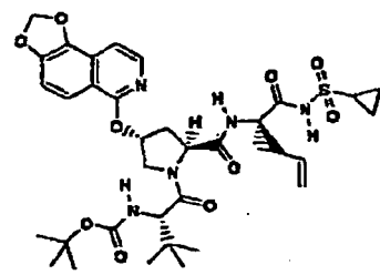
Composé 211 ;
