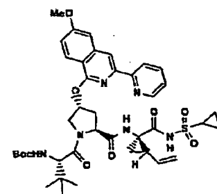
Composé 320 ;
