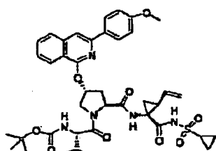
Verbindung 25
