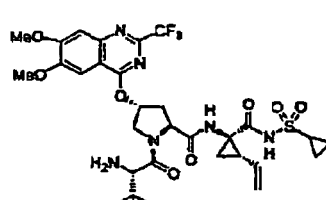
Composé 52
