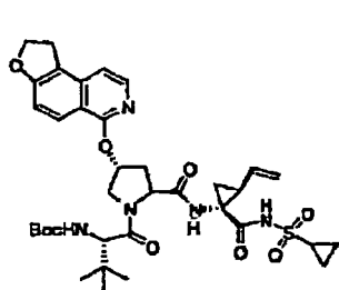
Verbindung 267
