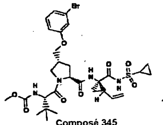
Composé 345
