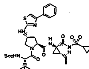
Verbindung 53
