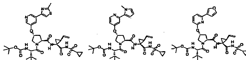
Verbindung 433
