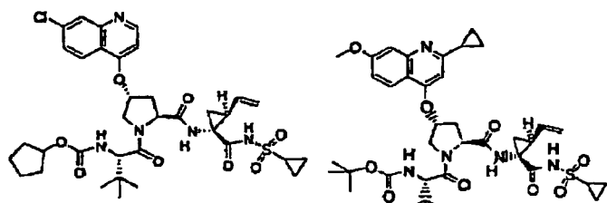
Verbindung 372
