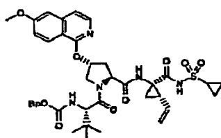
Verbindung 64
