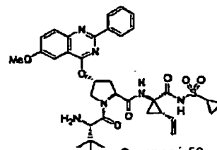
Composé 50
