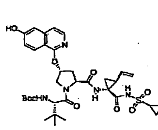
Verbindung 280
