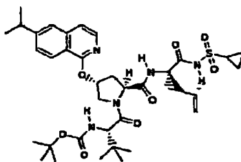
Verbindung 190
