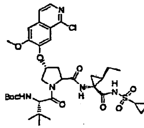
Verbindung 300
