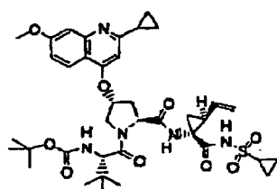
Composé 373 ;
