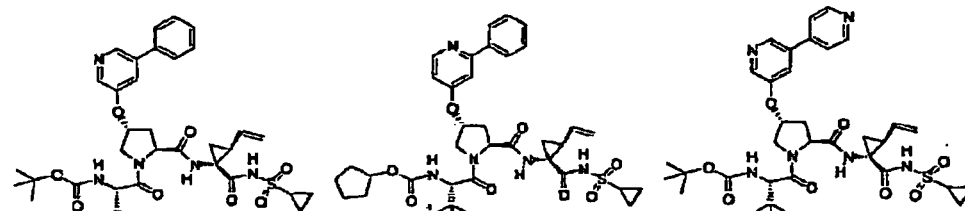
Composé 421 ;
