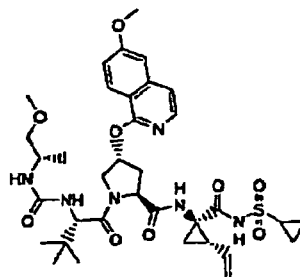
Composé 153
