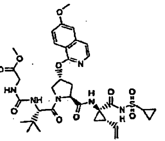
Composé 144
