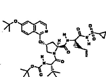
Verbindung 193
