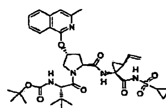
Verbindung 33
