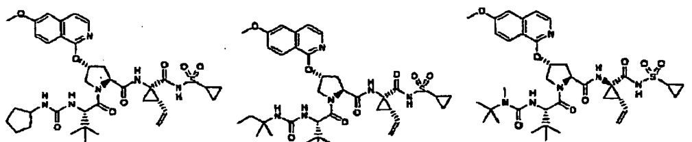
Verbindung 75
