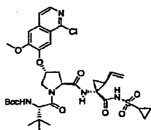
Verbindung 262
