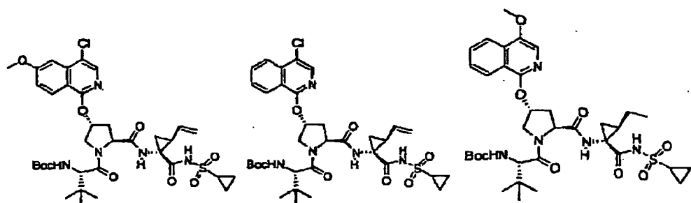
Verbindung 278
