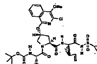
Verbindung 245
