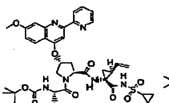
Composé 379 ;
