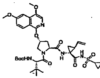
Verbindung 279
