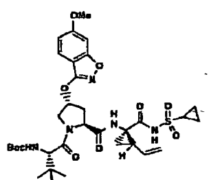
Verbindung 323
