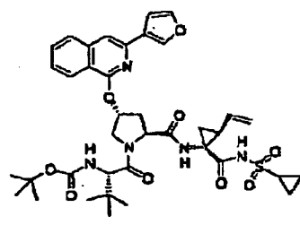
Verbindung 30
