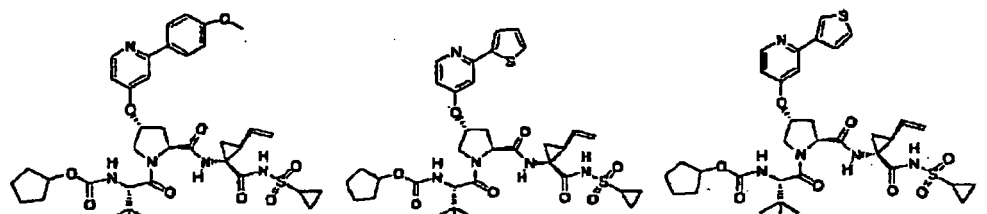
Verbindung 428
