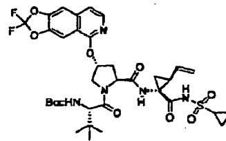
Composé 288 ;
