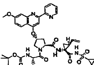
Verbindung 379
