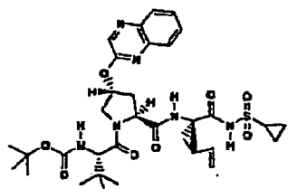
Verbindung 237
