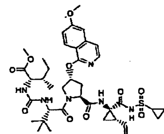
Verbindung 151
