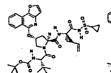
Verbindung 220
