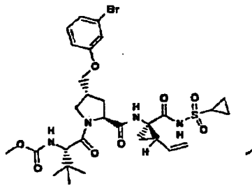
Verbindung 345
