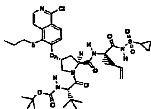
Composé 204
