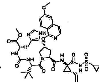
Verbindung 147
