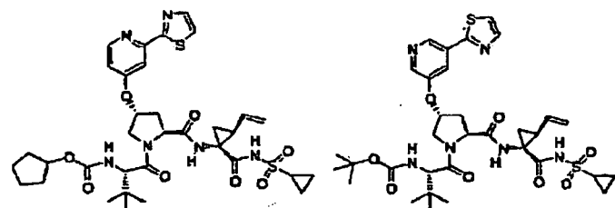
Verbindung 431
