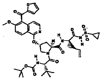
Composé 209 ;
