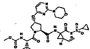
Verbindung 343
