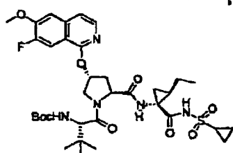
Verbindung 298
