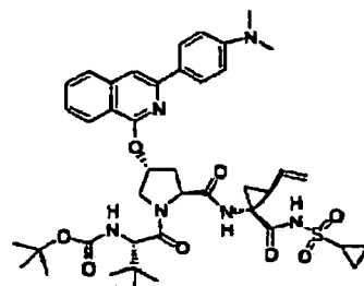
Verbindung 28
