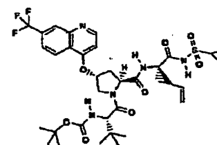
Composé 185
