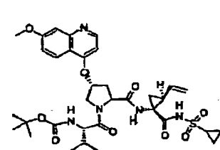
Verbindung 378
