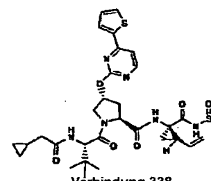
Verbindung 338
