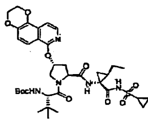
Composé 290 ;
