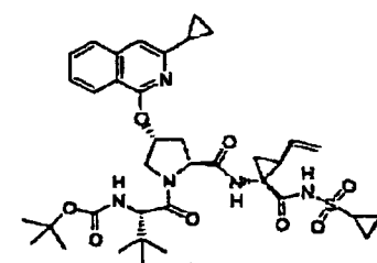
Verbindung 34
