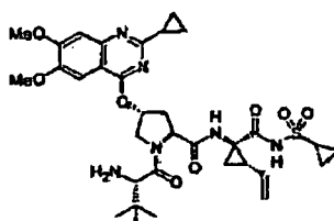
Composé 49
