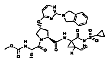
Verbindung 342
