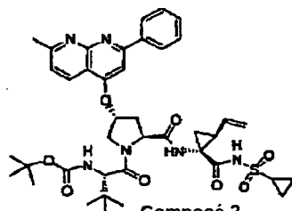
Composé 2
