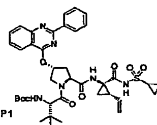
Composé 47
