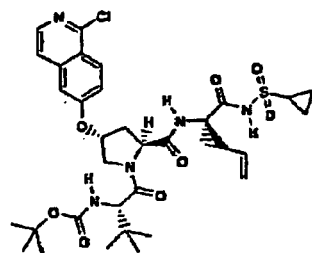
Composé 188
