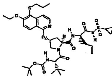
Verbindung 206
