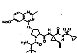
Composé 48
