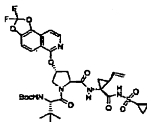
Composé 287 ;
