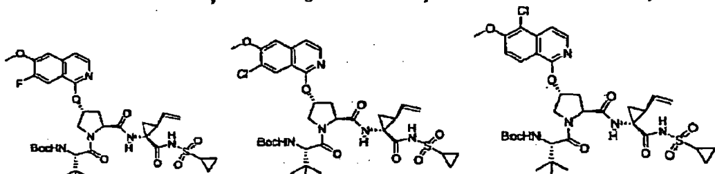
Verbindung 261
