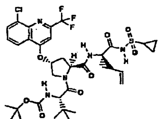
Composé 183
