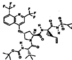
Composé 181
