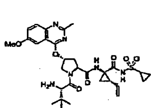
Verbindung 48
