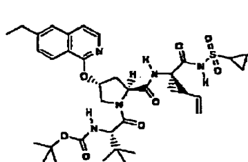
Verbindung 189
