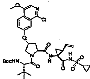
Verbindung 283
