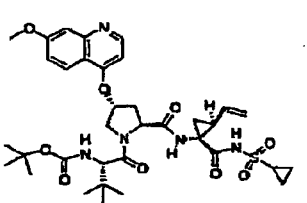
Composé 376 ;
