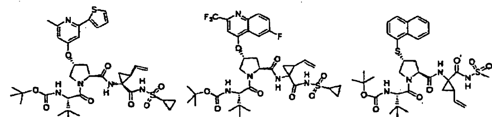
Verbindung 450
