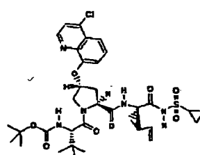
Composé 242
