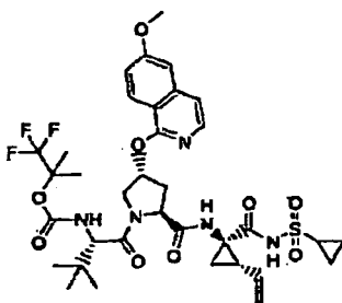
Composé 155
