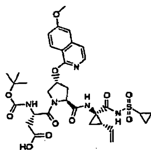
Composé 140
