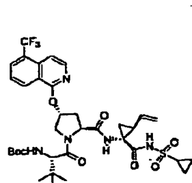
Verbindung 270
