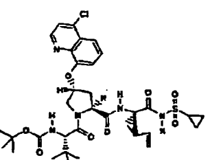
Verbindung 242
