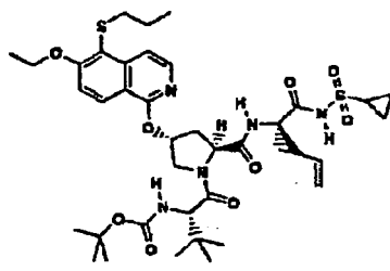
Composé 206 ;
