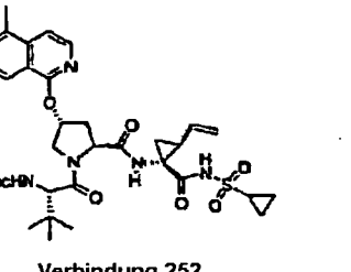
Verbindung 252
