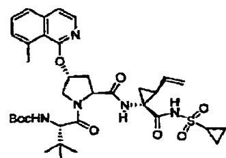
Composé 263 ;
