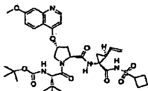
Composé 374 ;
