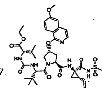
Composé 148
