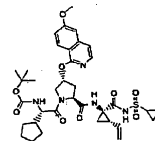
Composé 149
