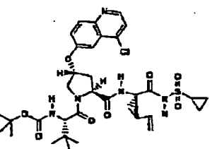
Verbindung 240
