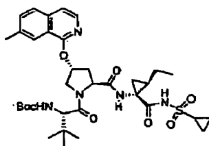
Composé 296 ;
