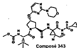
Composé 343
