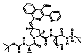
Verbindung 231
