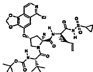
Verbindung 212
