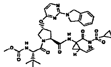
Verbindung 342
