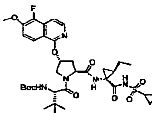
Verbindung 299
