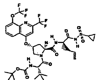
Verbindung 182
