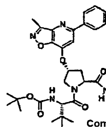
Composé 1
