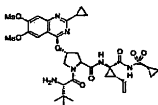
Verbindung 49
