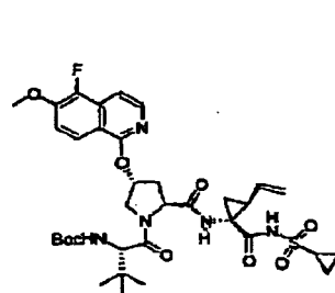
Verbindung 274
