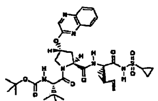
Composé 237
