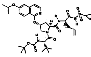
Composé 192
