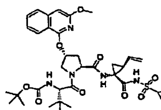
Verbindung 35
