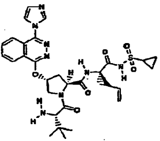
Composé 197
