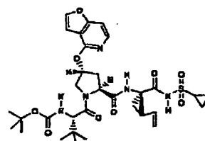
Composé 233
