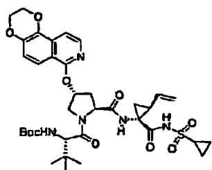
Composé 286 ;
