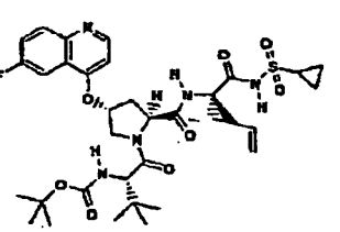
Verbindung 239
