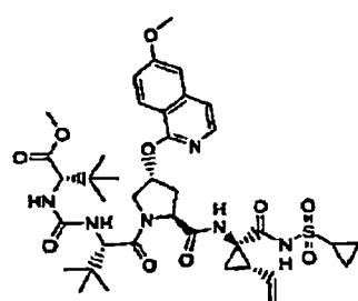
Verbindung 146
