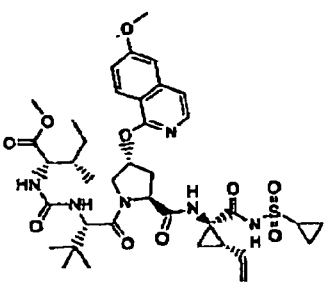
Composé 151
