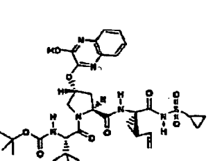
Verbindung 243
