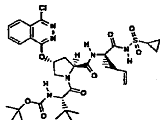
Composé 195
