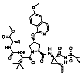
Verbindung 145
