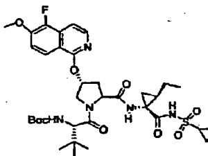
Composé 299 ;
