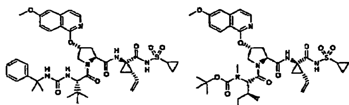
Verbindung 83
