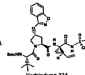
Verbindung 334
