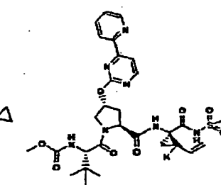
Verbindung 336
