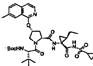
Verbindung 296
