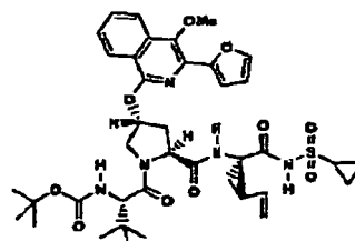
Verbindung 230
