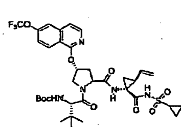
Verbindung 282
