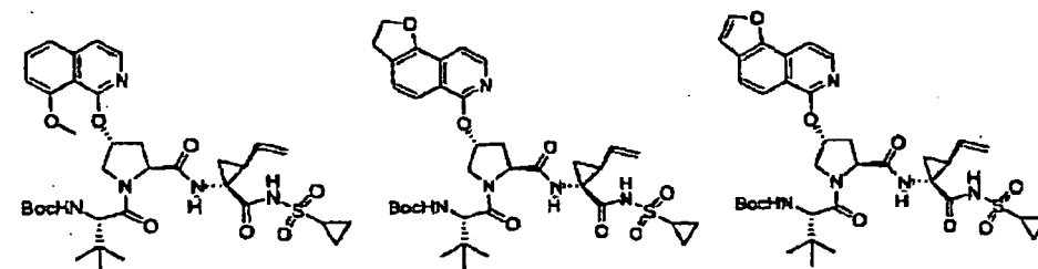
Composé 266 ;
