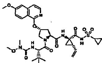
Composé 78
