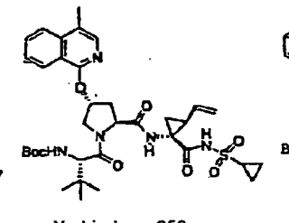
Verbindung 250
