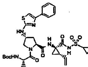
Composé 53
