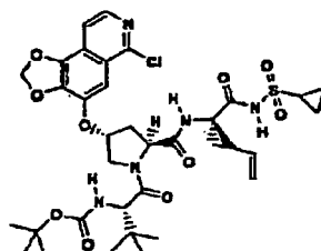
Composé 212
