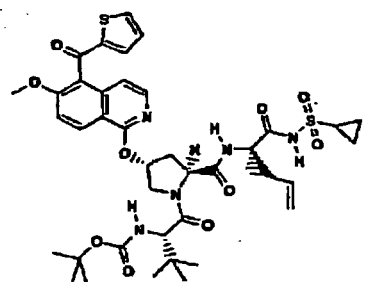
Verbindung 209
