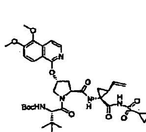
Verbindung 272
