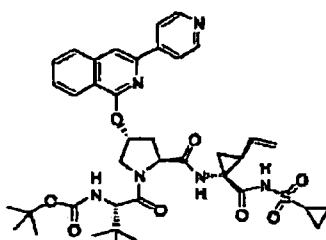
Verbindung 27
