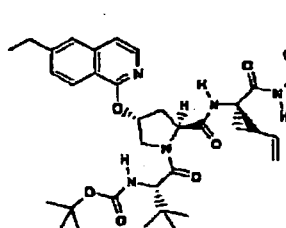
Composé 189
