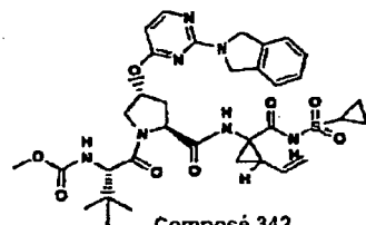
Composé 342
