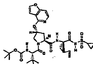
Verbindung 233
