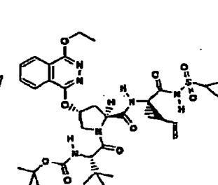
Composé 200
