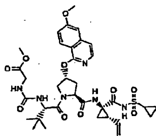
Verbindung 144
