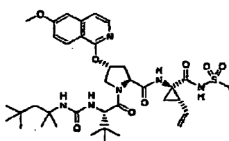
Composé 81
