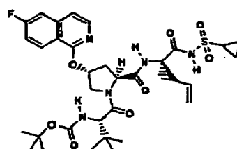
Verbindung 187
