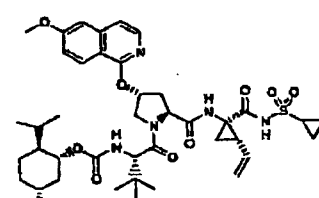
Verbindung 66
