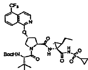
Composé 295 ;
