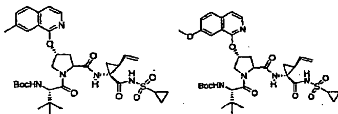
Composé 260 ;
