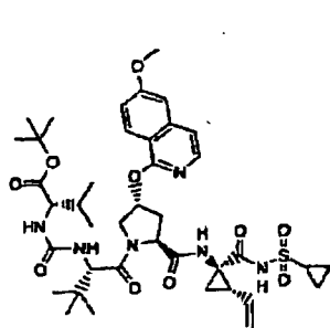
Composé 152
