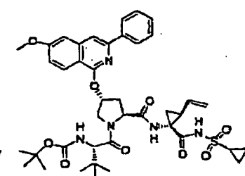
Verbindung 36
