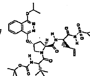
Composé 199
