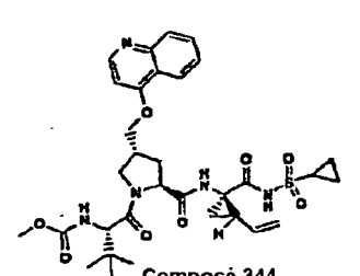
Composé 344
