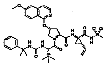
Composé 83
