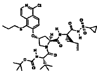
Verbindung 204
