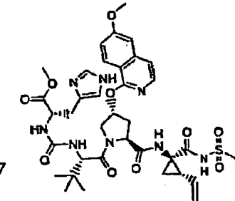
Composé 147
