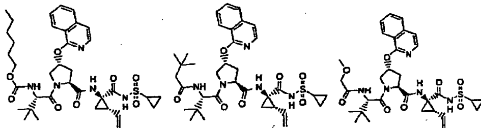
Verbindung 131
