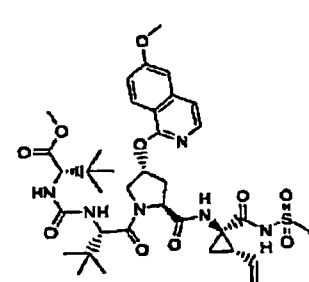
Composé 146
