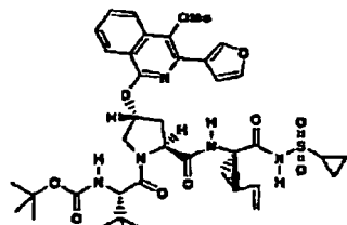
Verbindung 229
