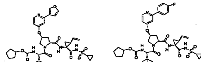
Composé 426 ;
