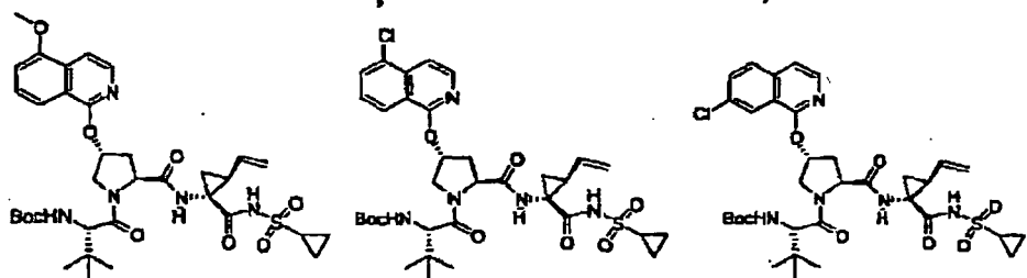
Verbindung 258
