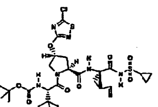
Verbindung 236
