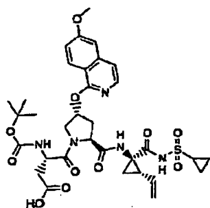
Verbindung 140
