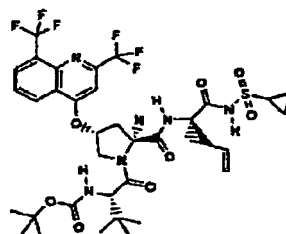
Verbindung 181
