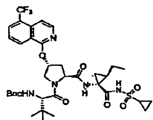
Verbindung 295
