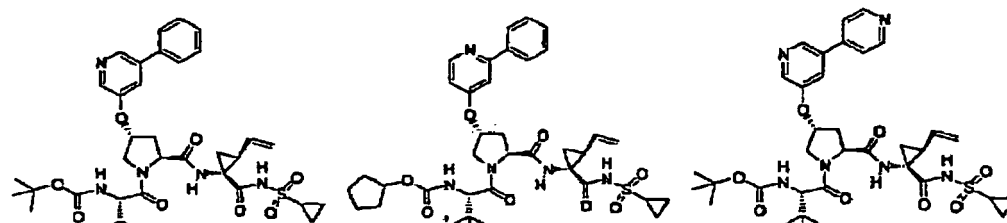
Verbindung 421
