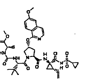
Composé 145
