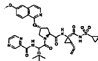
Verbindung 63
