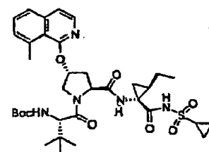
Verbindung 297
