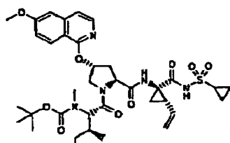
Composé 84
