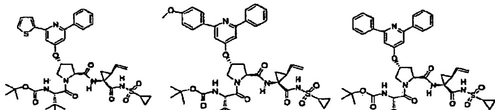
Verbindung 415
