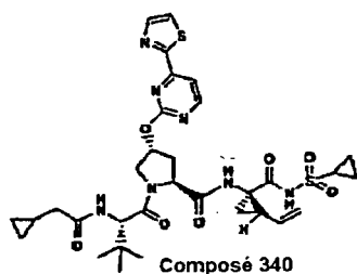
Composé 340
