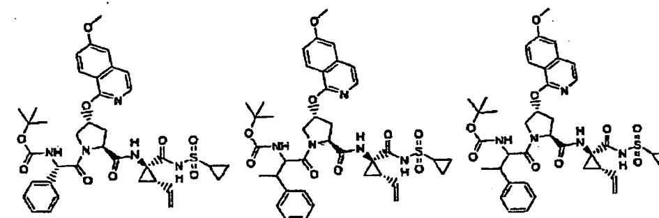
Verbindung 136
