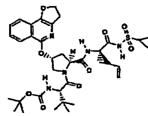
Verbindung 219
