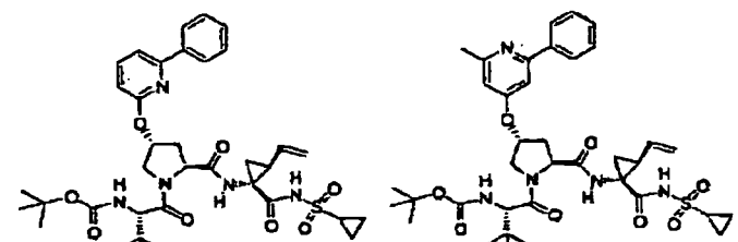
Verbindung 436
