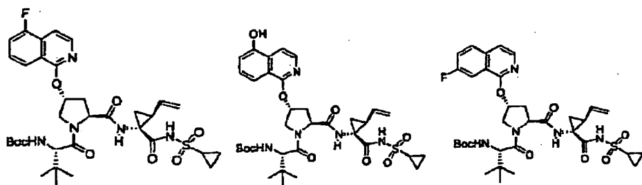
Composé 257 ;
