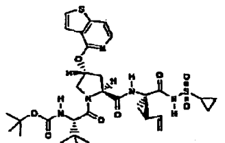
Verbindung 235
