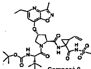
Composé 9
