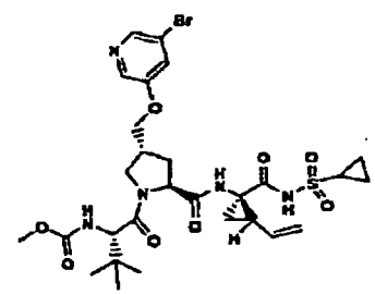
Verbindung 346
