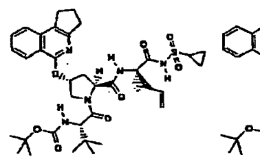
Verbindung 215
