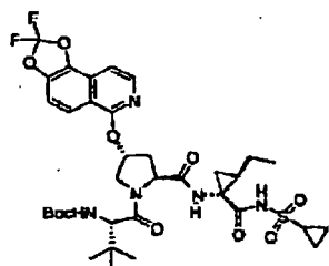
Verbindung 289
