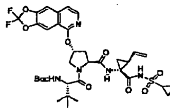
Verbindung 288
