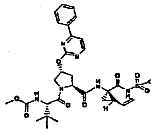
Verbindung 335
