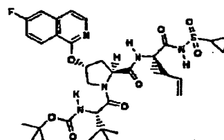
Composé 187
