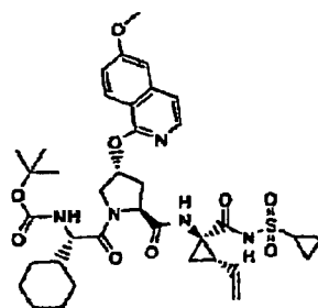
Verbindung 143
