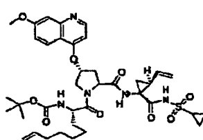
Composé 377 ;
