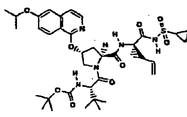
Verbindung 192
