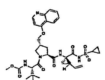
Verbindung 344
