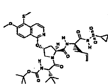
Verbindung 207
