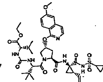
Verbindung 148
