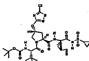
Composé 236
