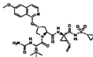
Composé 80
