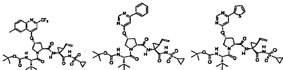
Verbindung 410
