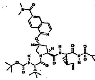
Verbindung 244
