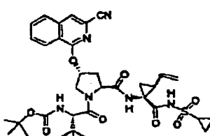
Verbindung 32
