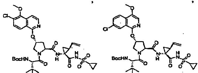
Verbindung 276
