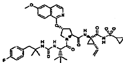
Composé 82
