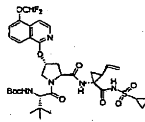
Verbindung 285
