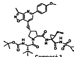
Composé 3
