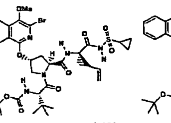
Composé 223 ;
