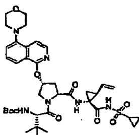
Verbindung 271
