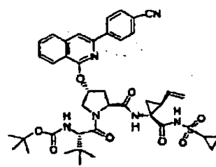
Verbindung 29
