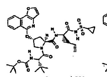
Composé 220 ;
