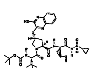
Composé 243
