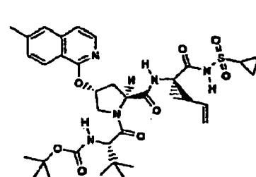
Verbindung 210
