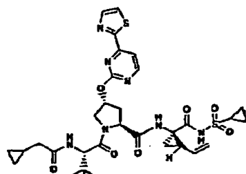
Verbindung 340
