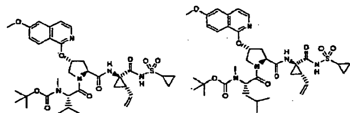
Verbindung 86
