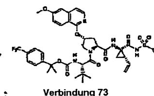
Verbindung 73
