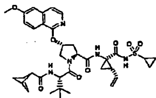
Verbindung 62
