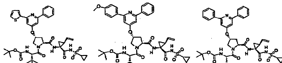
Composé 415 ;
