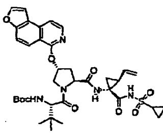
Verbindung 268
