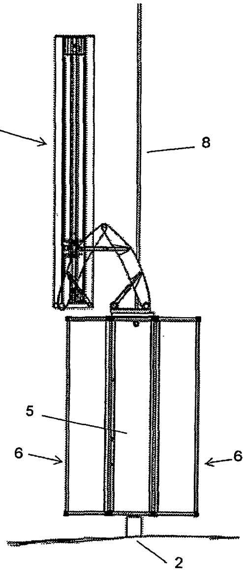
Fig. 3 Side elevation
