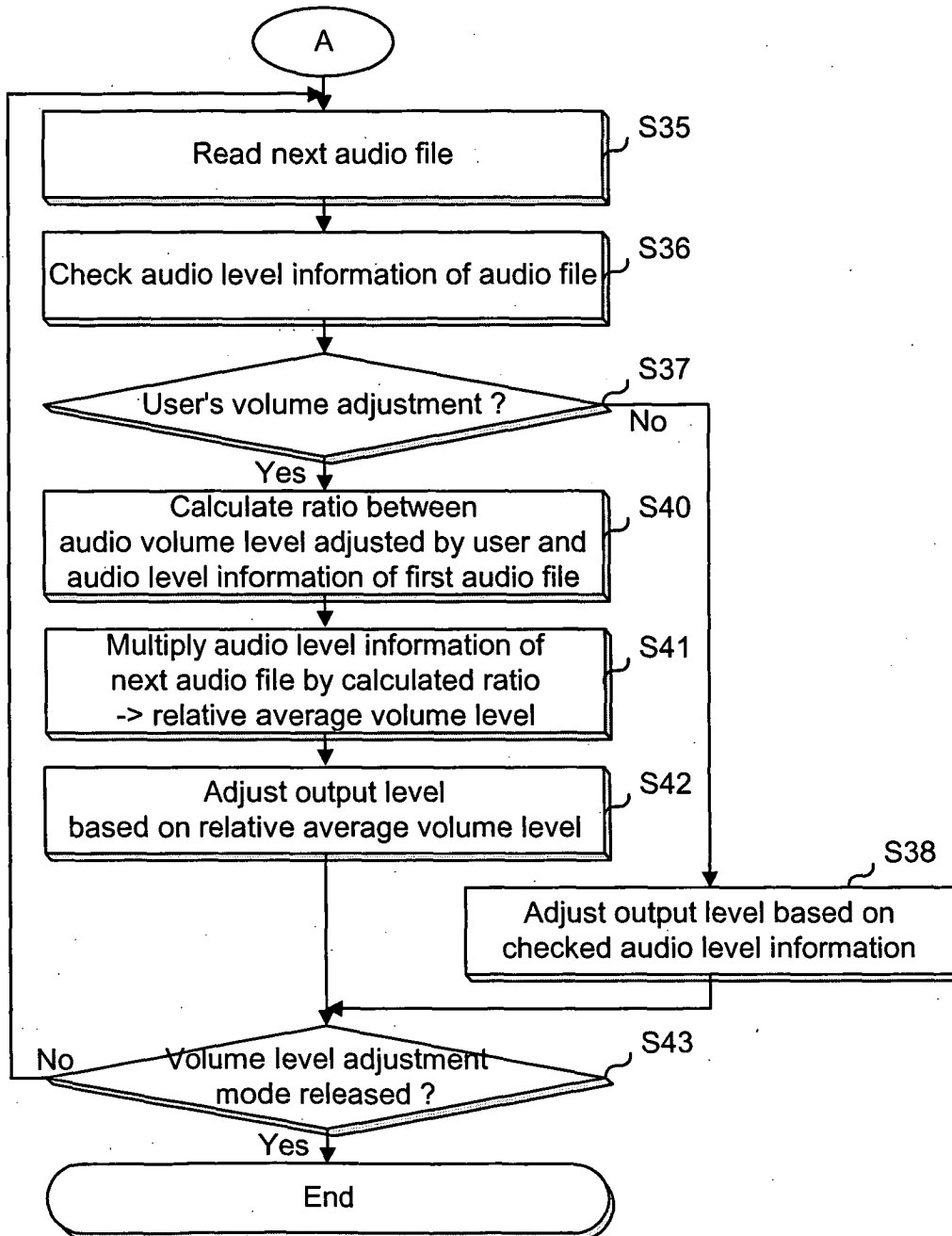
FIG. 7(b)
