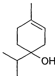
terpinen-4-ol
