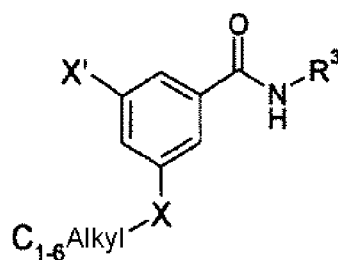
Formel (IIIe)
