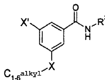
Formule (IIIe)
