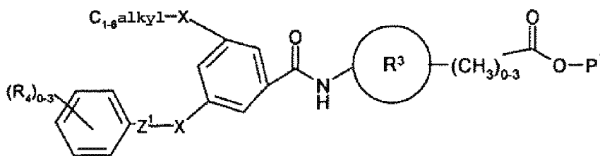
Formule (IIIc)
