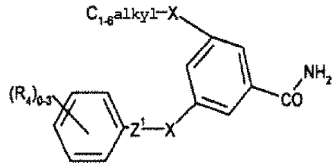
Formule (IIIIf)
