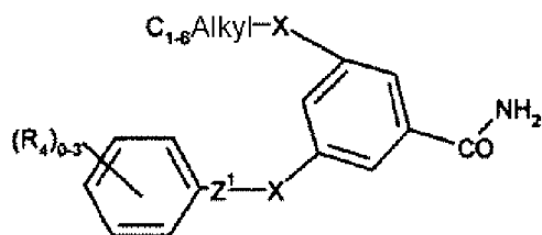
Formel (IIIIf)
