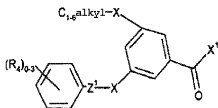
Formule (IIIa)
