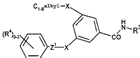
Formule (IIb)
