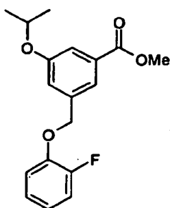
Compound (d)
