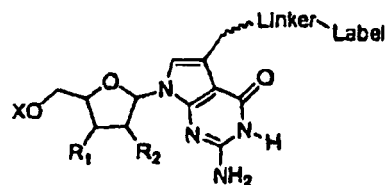
N7 Deazaguanosine C7-linker
