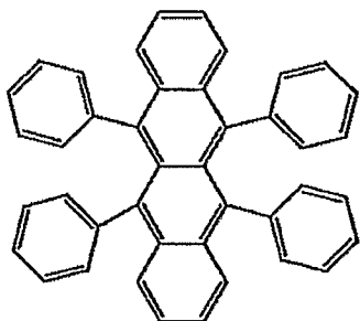
Rubrene
