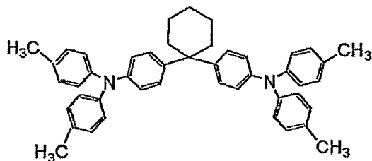
TPAC
