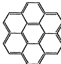
Coronene
