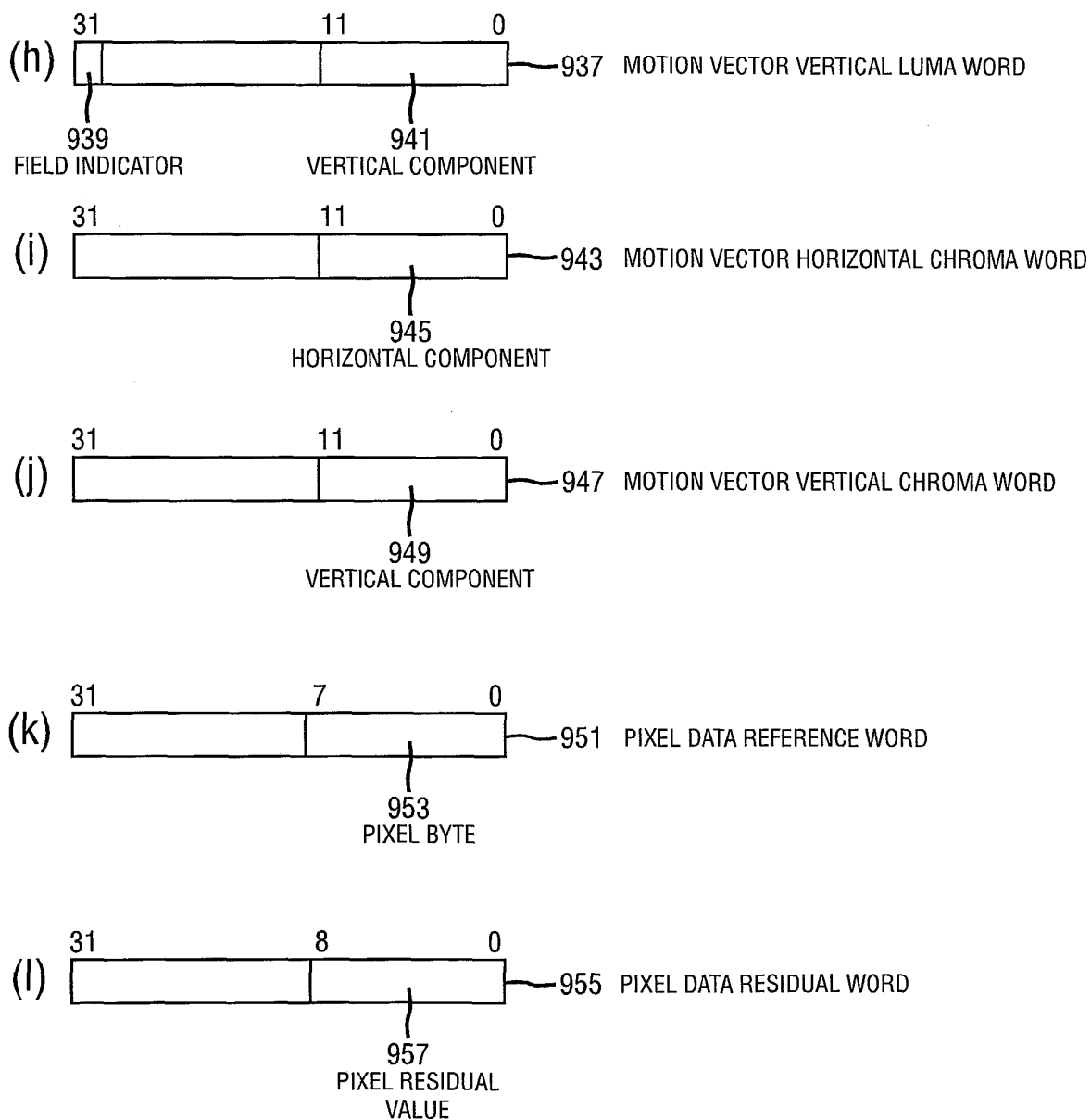
FIG. 9 (Contd.)
