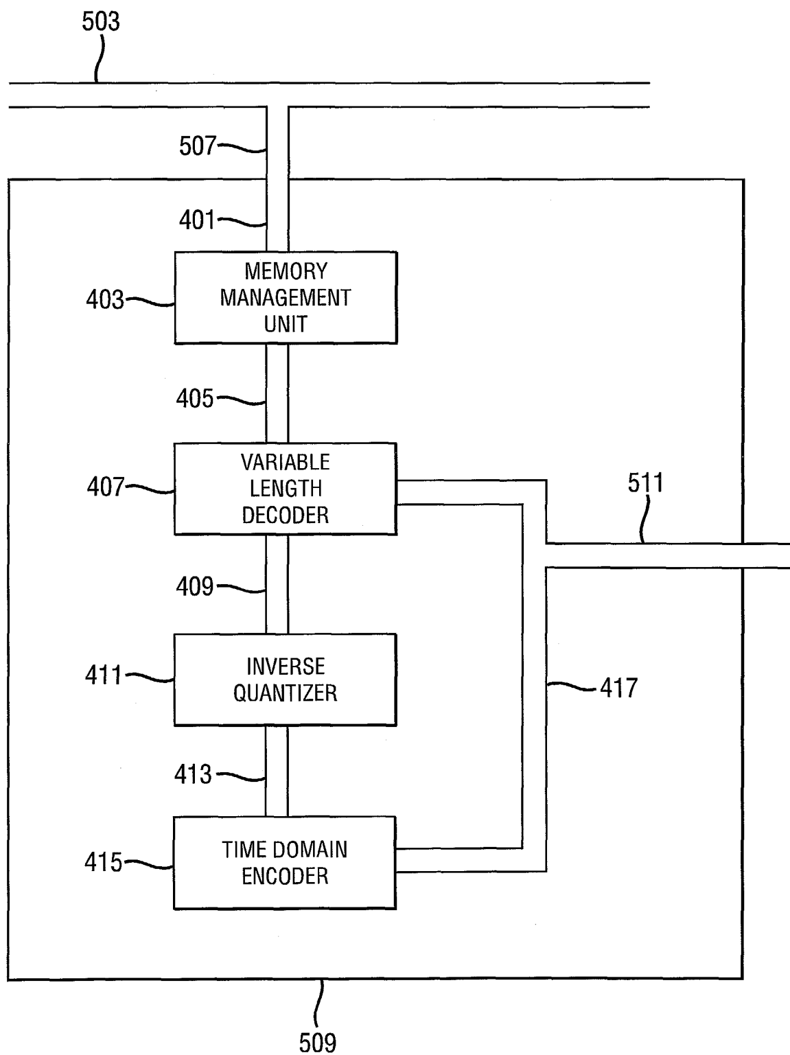
FIG. 5C
