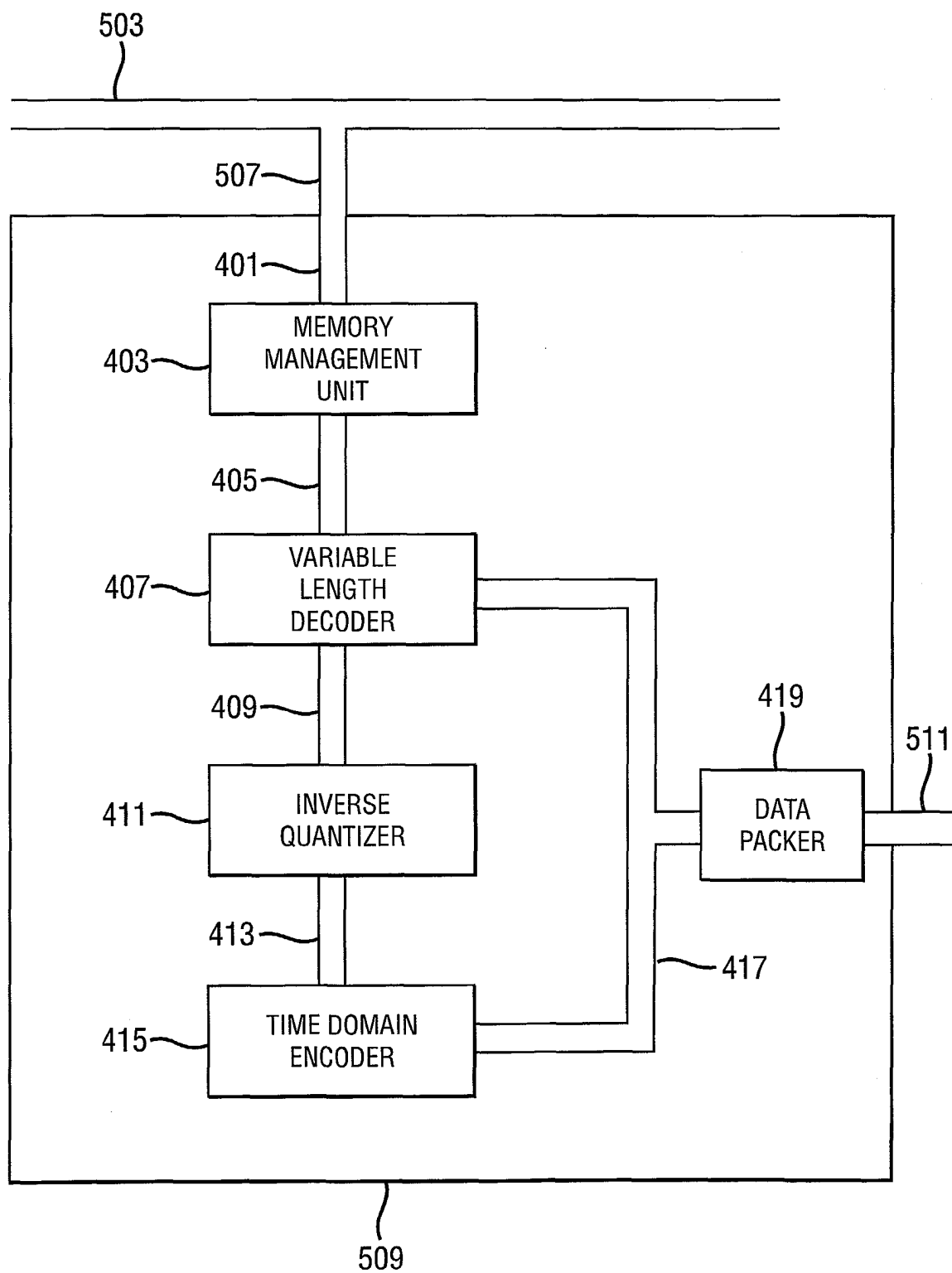
FIG. 5D
