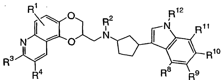
1a
