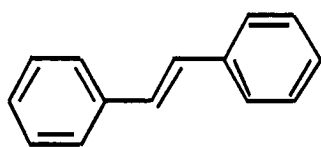
trans-stilbene
