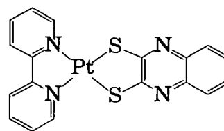
Pt(bpy)(qdt)
