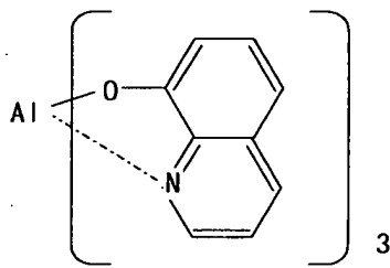
Alq
