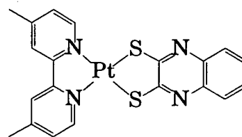
Pt(4dmbpy)(qdt)
