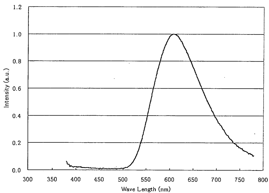
Pt(dpphen)(qdt) PL spectrum
