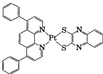
Pt(dpphen)(qdt)
