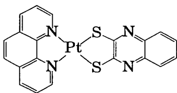
Pt(phen)(qdt)
