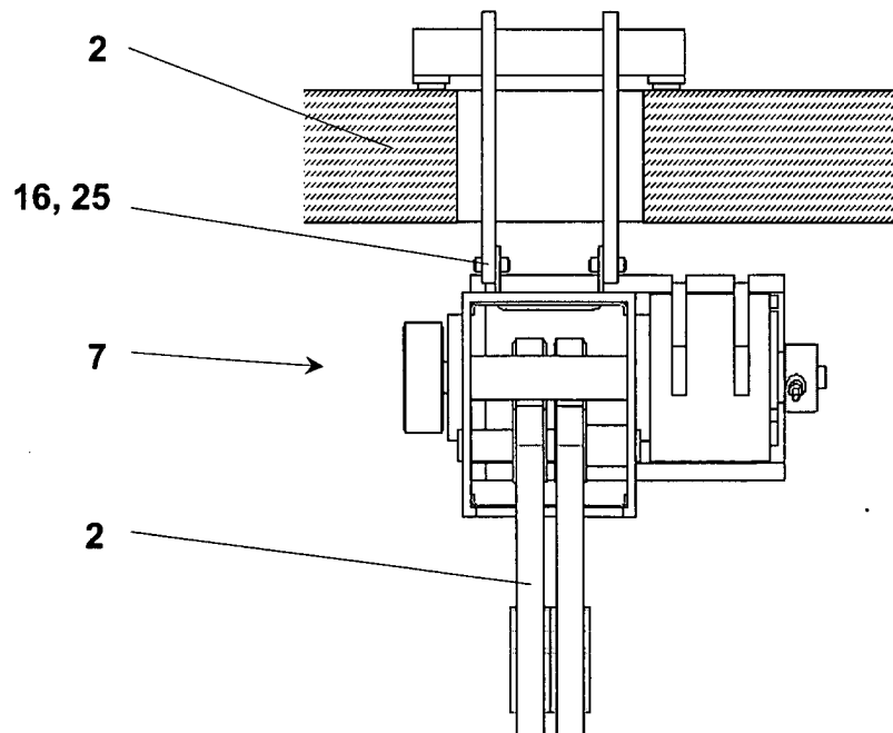
Fig. 8 A - A
