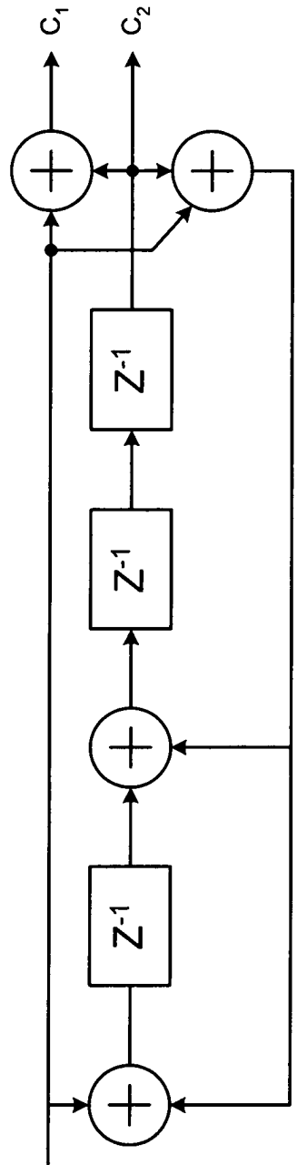
FIG. 12 channel encoder 174 (turbo encoder)
