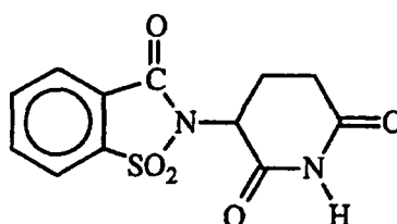
supidimide.
