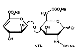
ΔIIsgal
