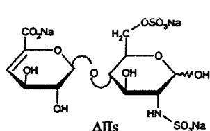
ΔIIs
