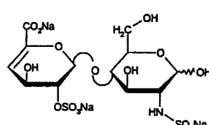
ΔIIIs
