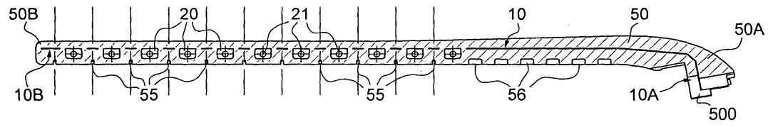
Fig. 2b COUPE A-A
