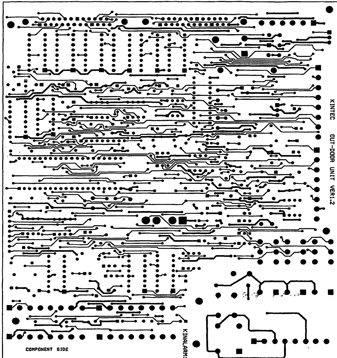
P.C.B. Top Side
